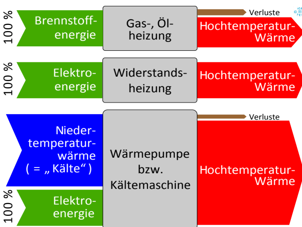
Energieflussdiagramme verschiedener Wärmeerzeuger
