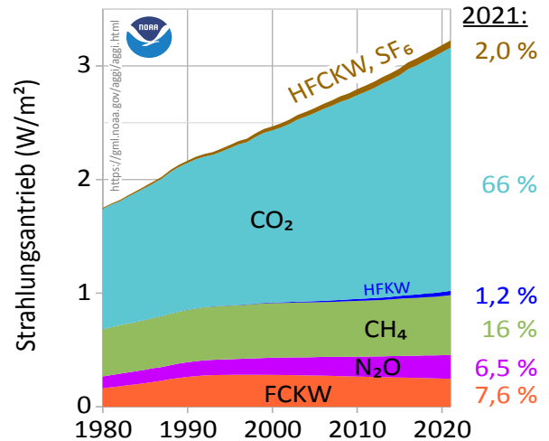
Treibhauswirksamkeit aller Treibhausgase
