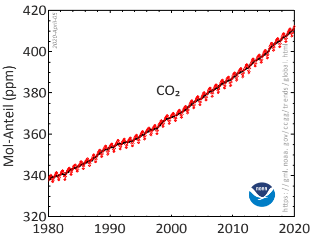
Globale CO 2 -Konzentrationen
