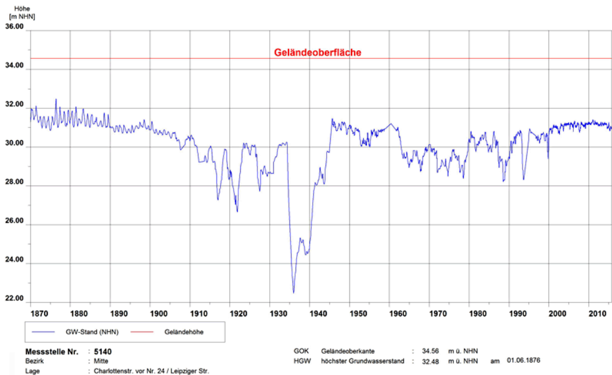
Abb. 9: Grundwasserstandsganglinie einer Messstelle aus der Innenstadt seit 1870. Der höchste Grundwasserstand (HGW) wurde hier am 1.6.1876 gemessen. Der Grundwasserstand ist durch zahlreiche Grundwasserabsenkungen seit 1905 zeitweise stark beeinflusst.
