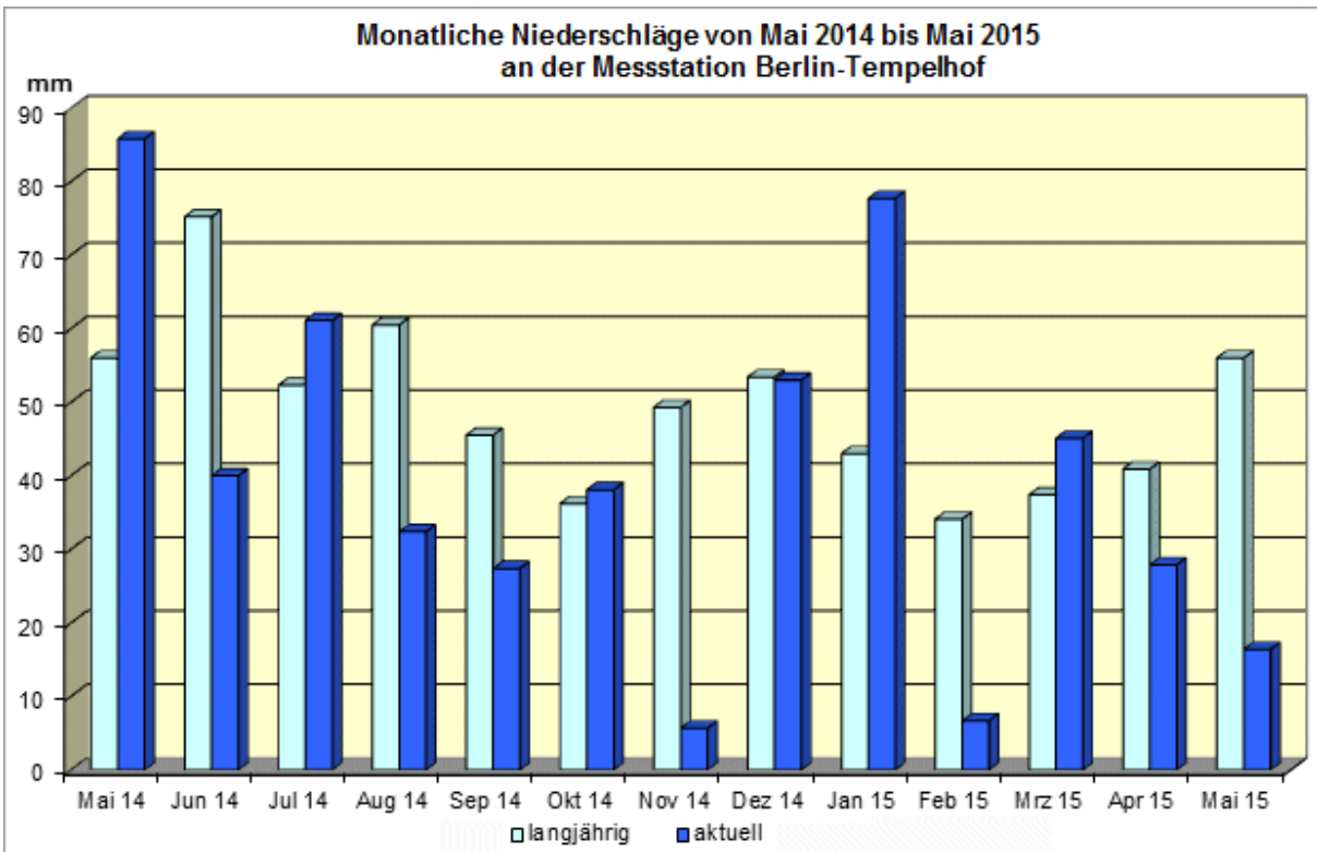
Abb. 15: Monatlicher Niederschlag von Mai 2014 bis Mai 2015 der Messstation Berlin-Tempelhof im Vergleich mit dem langjährigen Mittel 1961 bis 1990
