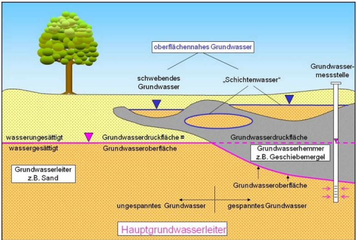
Abb. 3: Hydrogeologische Begriffe
