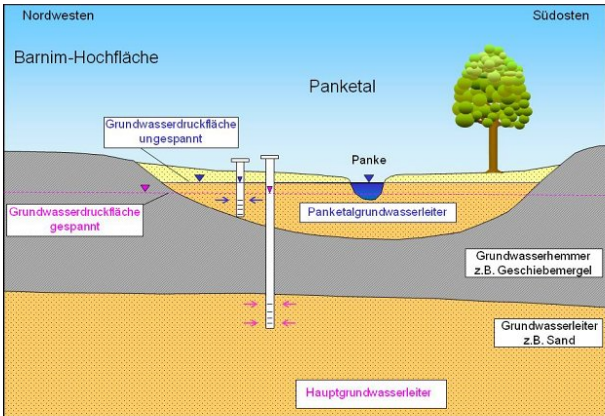
Abb. 8 Der ungespannte Panketalgrundwasserleiter (GWL 1) im nordwestlichen Bereich der Barnim-Hochfläche liegt über dem Hauptgrundwasserleiter (GWL 2), der hier gespannt ausgebildet ist
