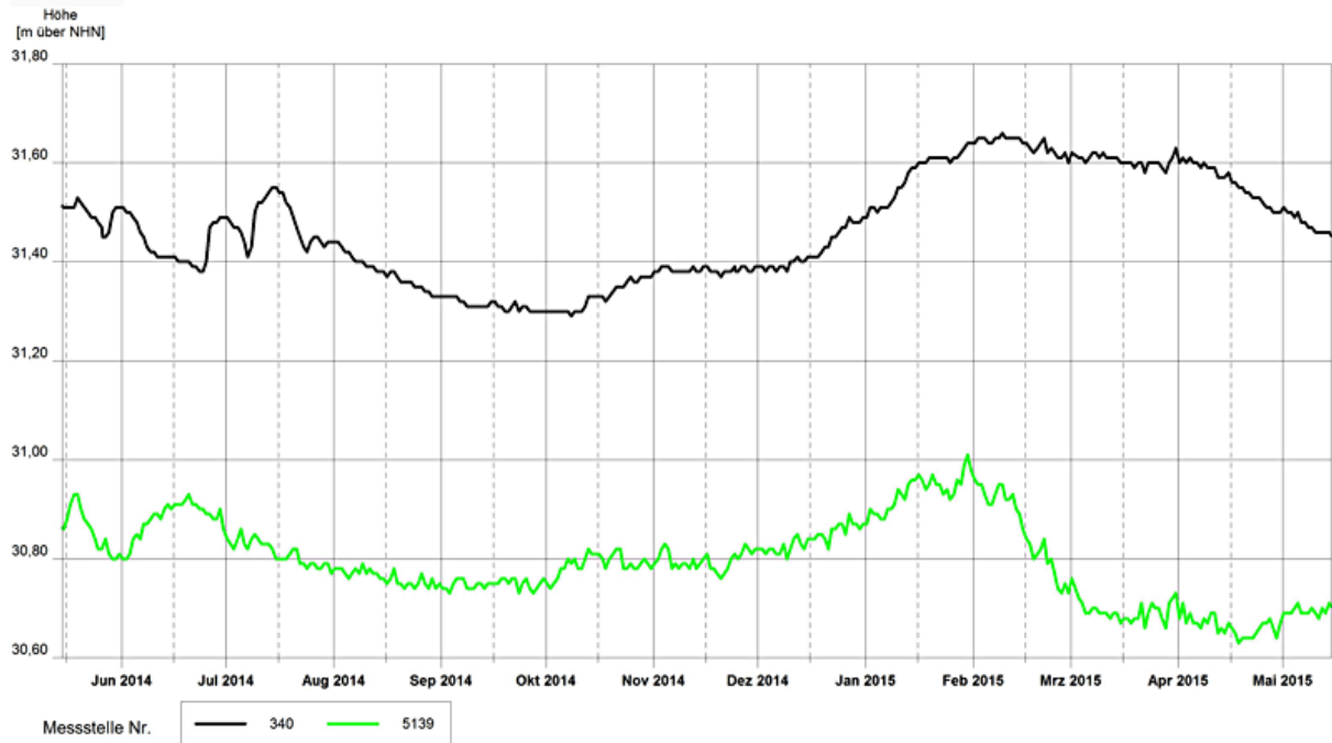
Abb. 13: Grundwasserstandsganglinien von zwei beispielhaften Messstellen im Urstromtal vom 15. Mai 2014 bis zum 15. Mai 2015
