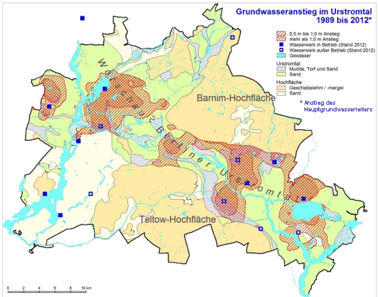
Abb. 10: Grundwasseranstieg von 1989 bis 2012 im Urstromtal
