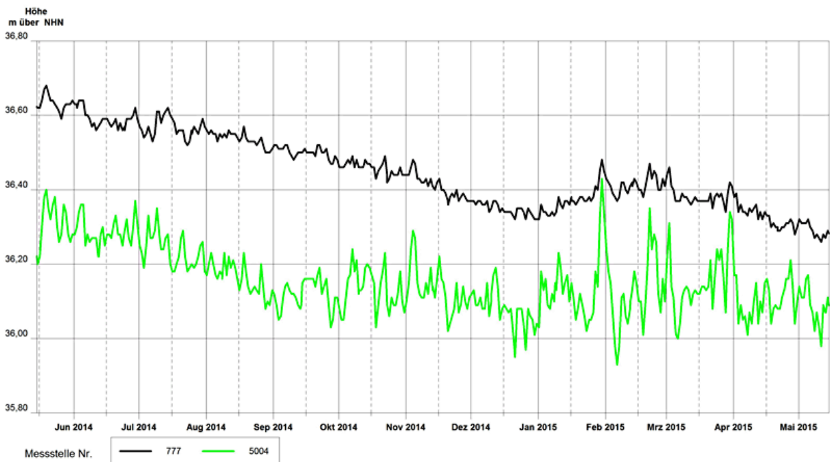
Abb. 14: Grundwasserstandsganglinien von zwei beispielhaften Messstellen auf den Hochflächen vom 15. Mai 2014 bis zum 15. Mai 2015
