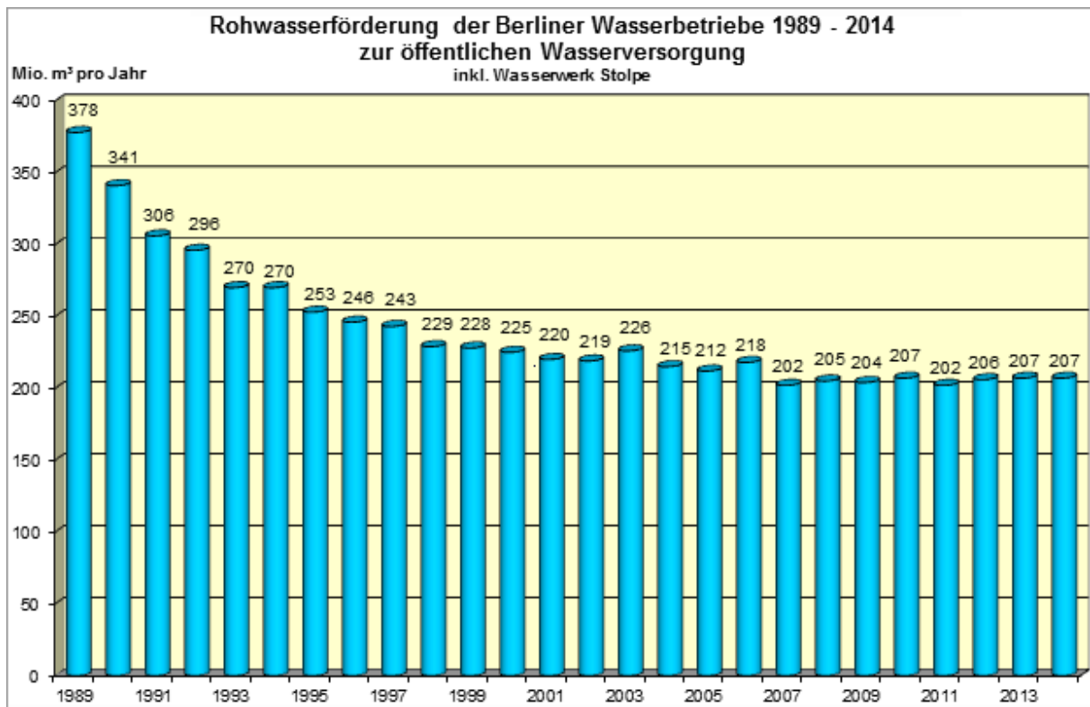
Abb. 11: Entwicklung der Rohwasserförderung der Berliner Wasserbetriebe in den letzten 26 Jahren
