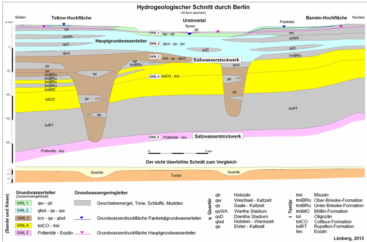
Abb. 7: Schematischer Hydrogeologischer Schnitt von Süden nach Norden durch Berlin
