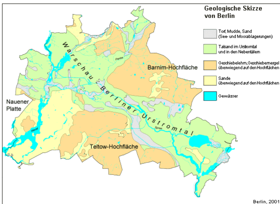
Abb. 6: Geologische Skizze von Berlin
