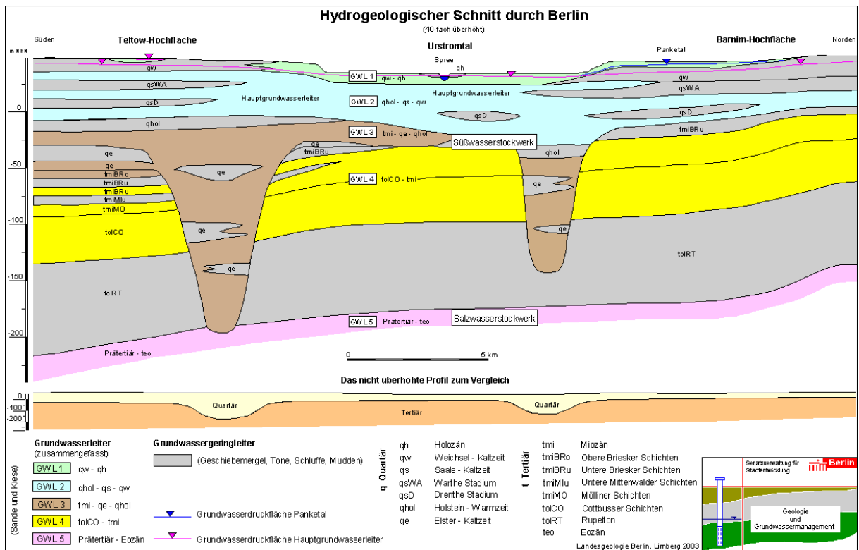
Abb. 7: Hydrogeologischer Schnitt durch Berlin
