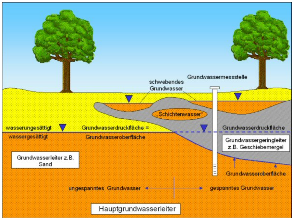
Abb. 3: Hydrogeologische Begriffe
