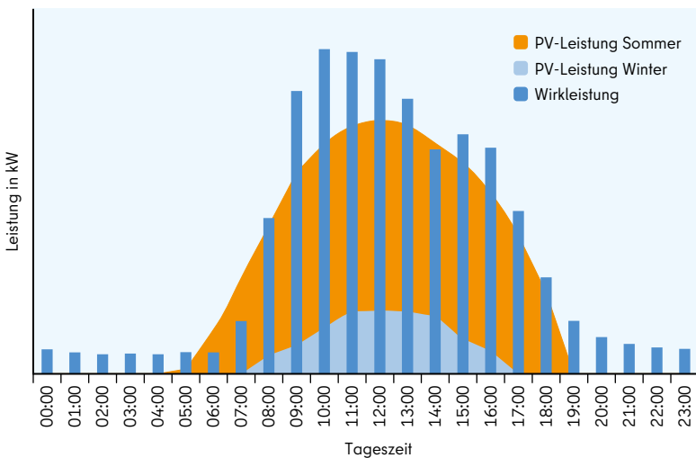
Abb. 1 | Zeitlicher Verlauf von PV-Erzeugung und Verbrauch
