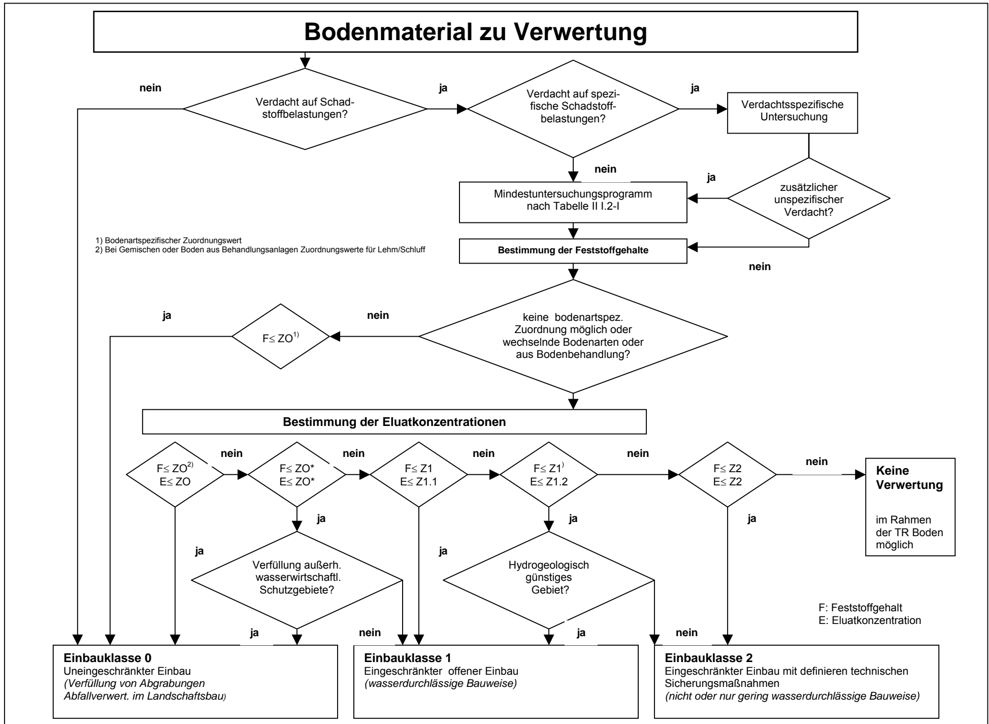
Flussbild: Verwertung von Bodenmaterial
