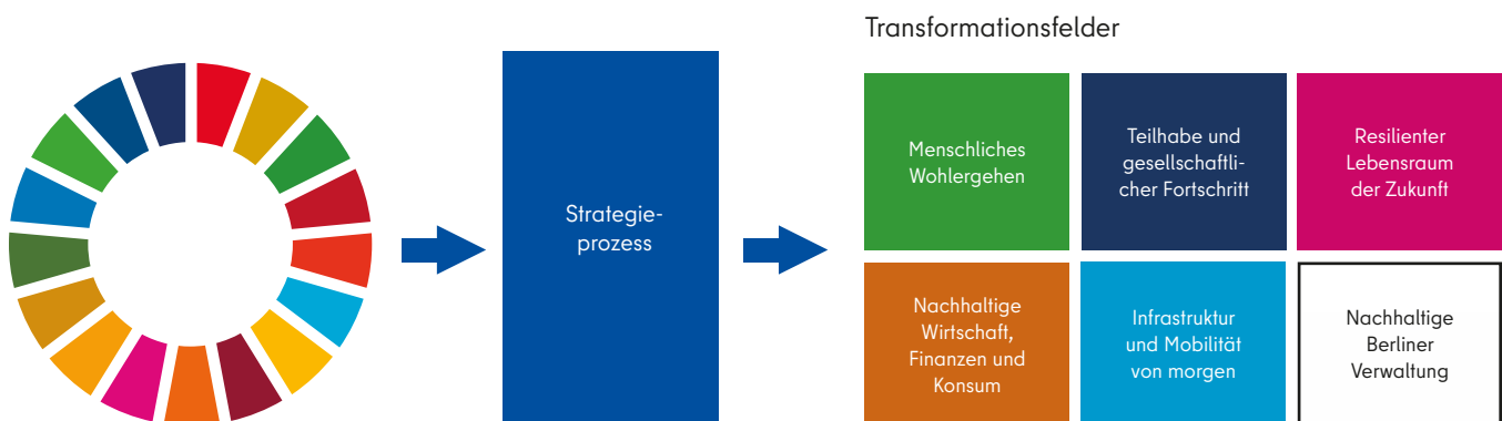
Abbildung 1: Entwicklungsprozess Transformationsfelder
