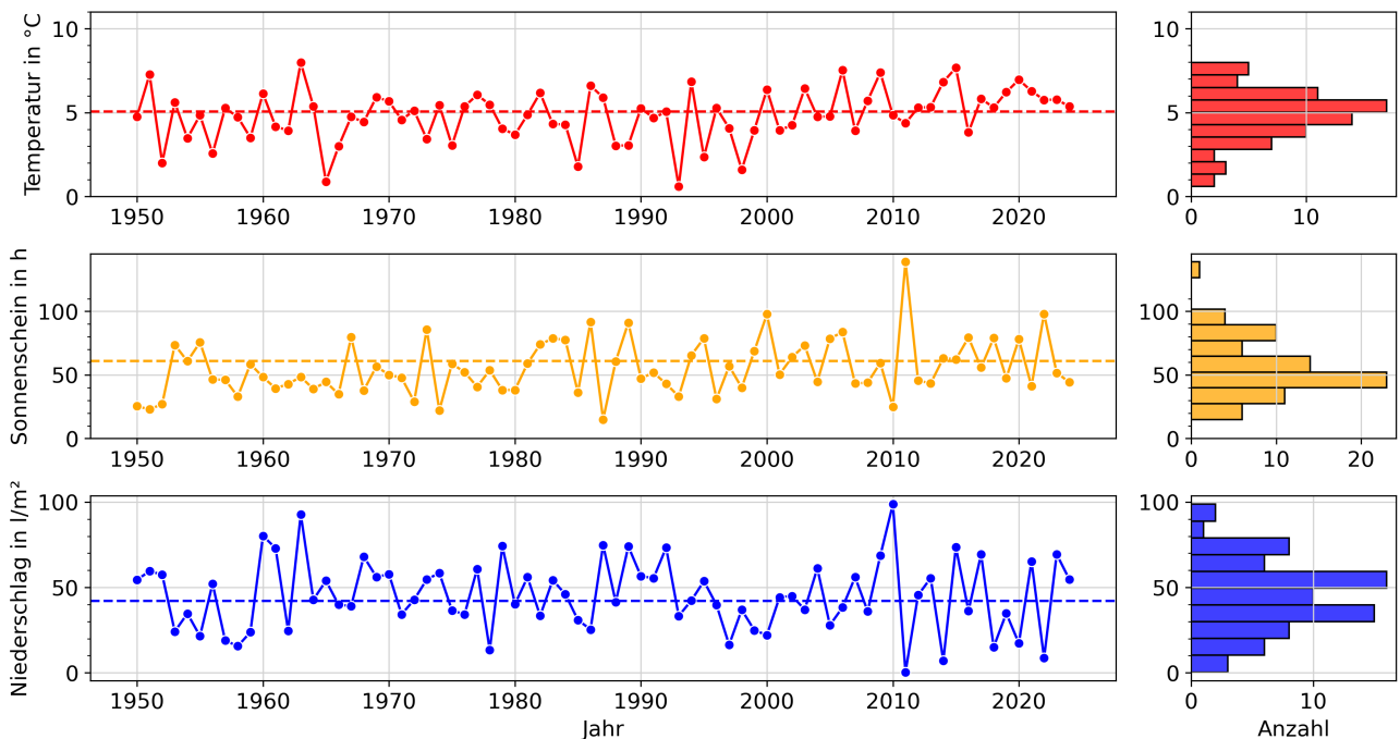
Abbildung 2: Mittelwerte für Temperatur, Sonnenscheindauer und Niederschlagsmenge im November 1950 bis 2024 für die DWD-Station Berlin-Dahlem. Die gestrichelten Linien zeigen die Mittelwerte der November-Monate von 1991 bis 2020. Die Histogramme rechts in der Abbildung veranschaulichen die Verteilungen dieser Parameter.
