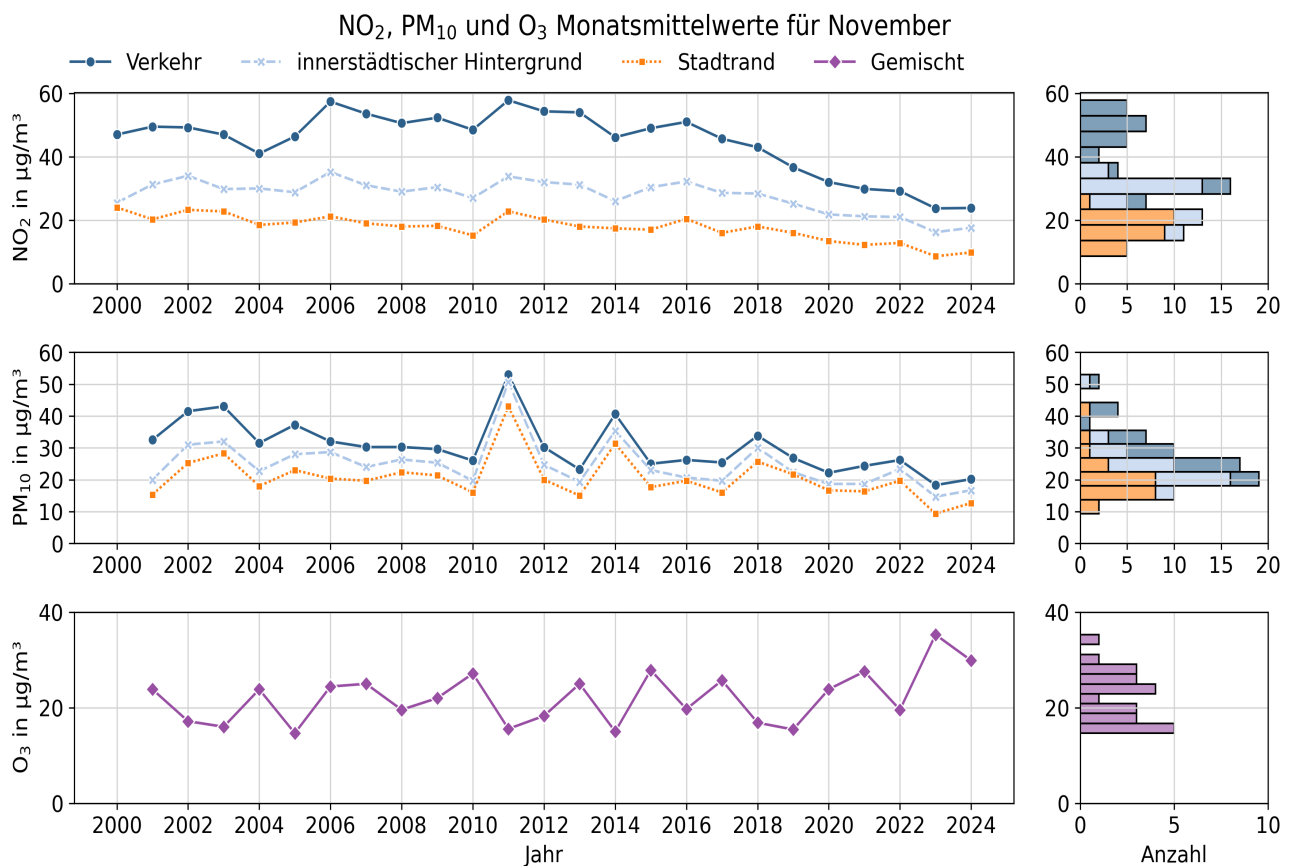
Abbildung 3: Zeitreihen der Monatsmittelwerte der Luftschadstoffe Stickstoffdioxid, PM 10 und Ozon zwischen 2000 und 2024, dargestellt für die Belastungsregime Straße, Innenstadt und Stadtrand. Die Ozonwerte basieren auf allen Stationen am Stadtrand und im innerstädtischen Hintergrund. Rechts sind die Verteilungen der Parameter als Histogramm dargestellt.
