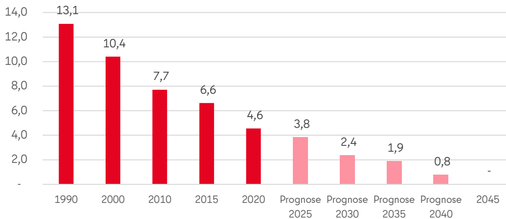
Entwicklung der CO 2 -Emissionen (Mio. Tonnen pro Jahr) der BEW Berliner Energie und Wärme GmbH (BEW), ab 2025 gemäß Planungsvorgaben
