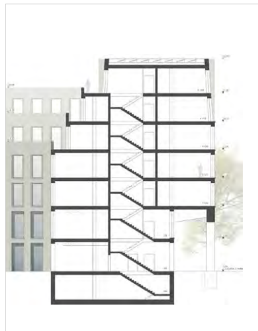
▲ Schnitt B3.2
