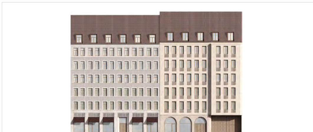
▲ Ansicht Jüdenstraße
