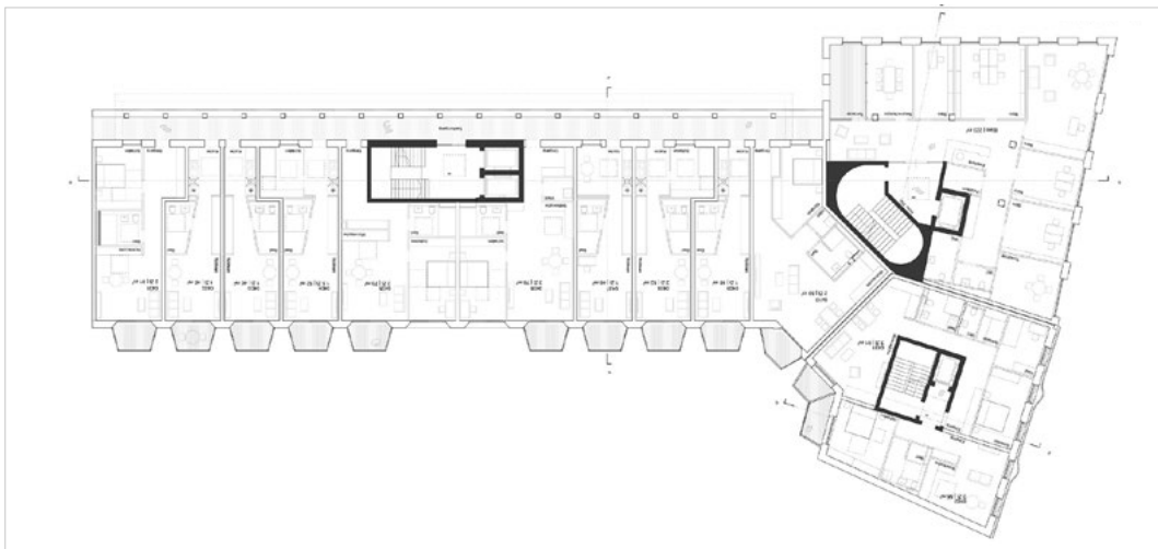
▲ Grundriss RG
