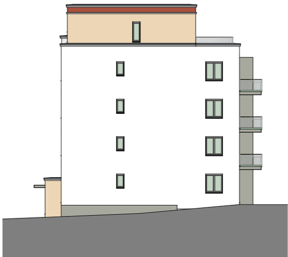
Haus b Ansicht West
