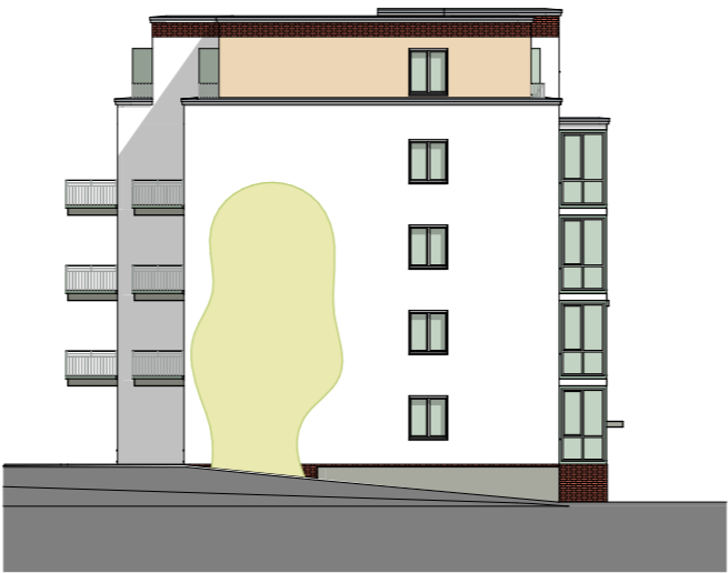
Haus a Ansicht Nord
