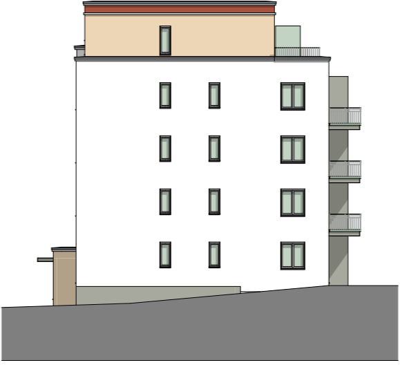
Häuser g // h Ansicht West
