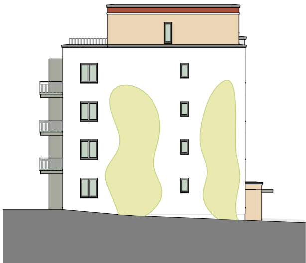
Haus b Ansicht Ost
