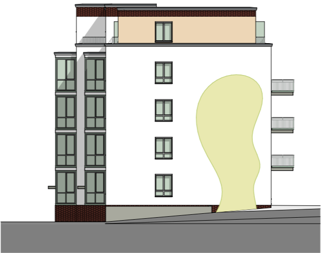
Haus a Ansicht Süd
