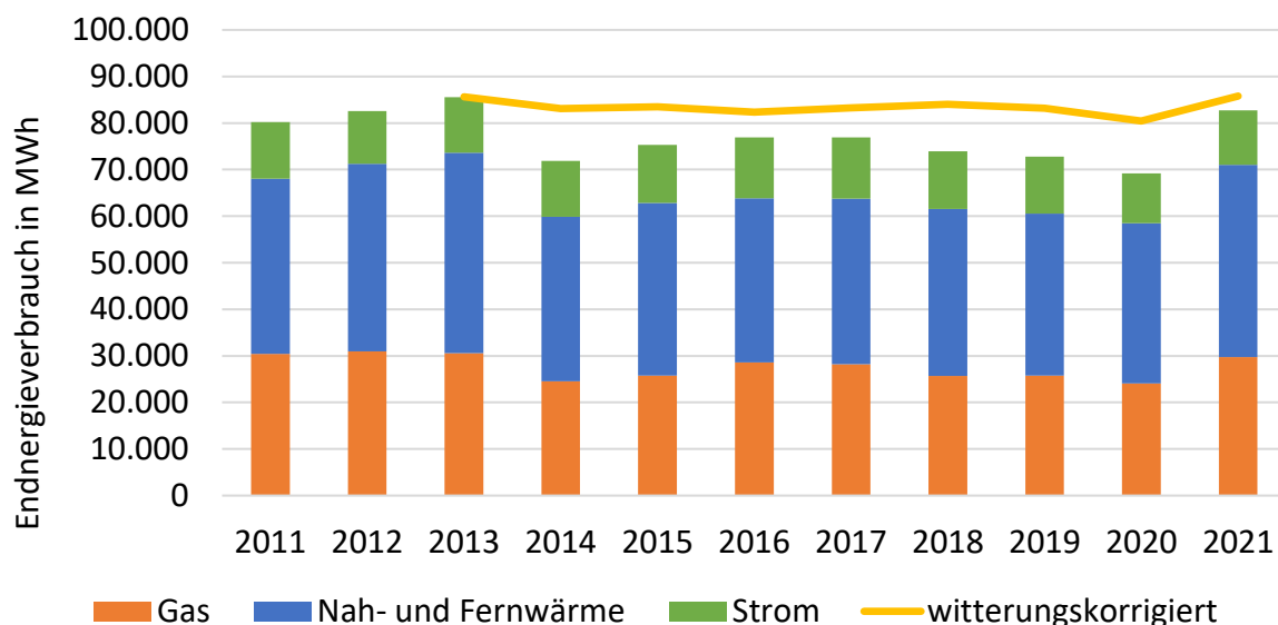
Abbildung 20: Energieverbrauch bezirklicher Gebäude 2011 - 2021. Quelle: Mellon, 2023
