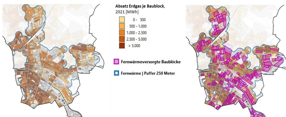
Abbildung 55: Potenziale für eine Nachverdichtung der Fernwärme im bestehenden Versorgungsgebiet. Quelle: Mellon, 2023
