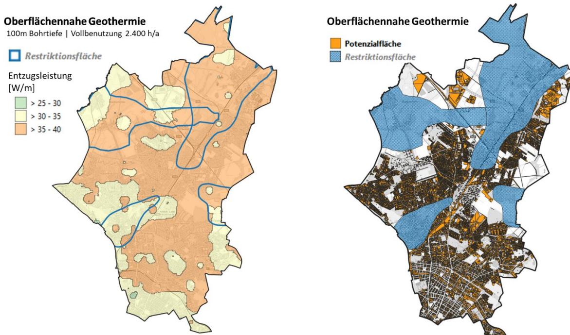
Abbildung 57: Restriktionsflächen, mögliche Entzugsleistungen und Annäherung an Potenzialfläche Oberflächennaher Geothermie. Quelle: Energieatlas Berlin, Darstellung von Mellon, 2023
