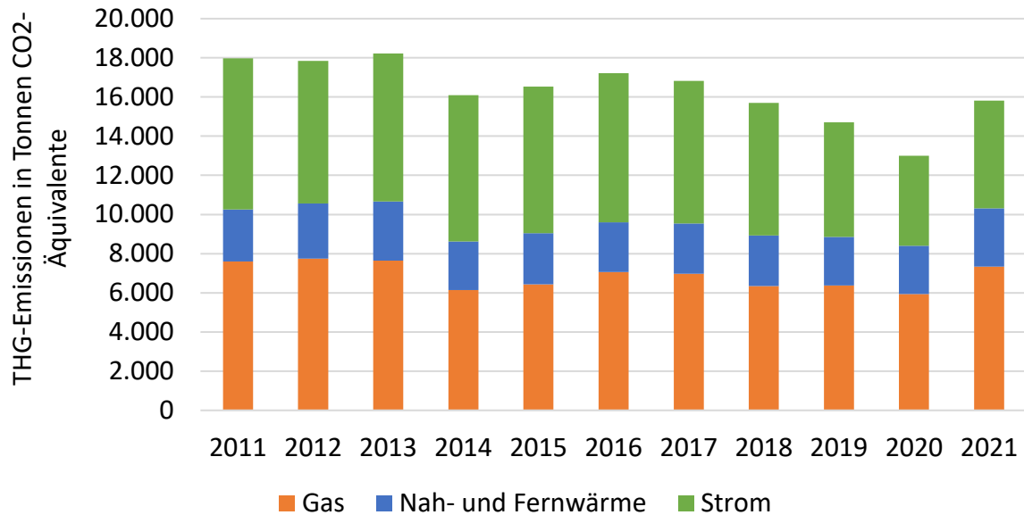
Abbildung 21: THG-Emissionen bezirklicher Gebäude, 2011 – 2021. Quelle: Mellon, 2023
