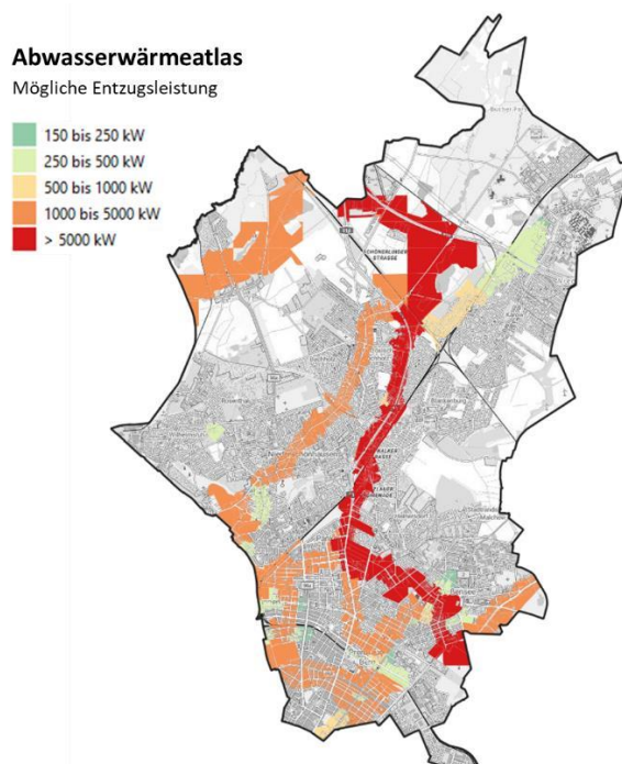
Abbildung 56: Mögliche Entzugsleistung aus dem Abwassernetz. Quelle: Abwasserwärmeatlas BWB, Darstellung von Mellon, 2023
