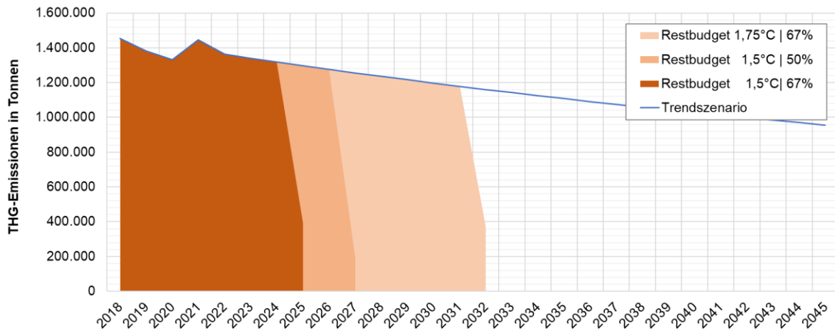
Abbildung 64: Lokales Trendszenario und Anwendung der Restbudgets. Quelle: Mellon, 2024
