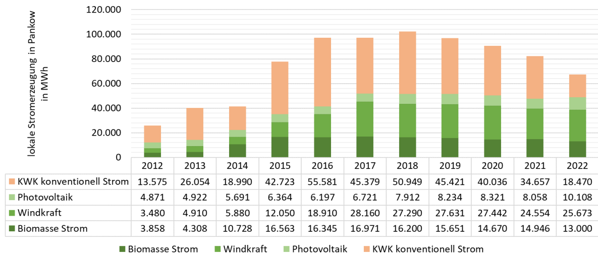
Abbildung 16: Verlauf und Anteile lokaler Stromerzeugung. Quelle: Mellon, 2023
