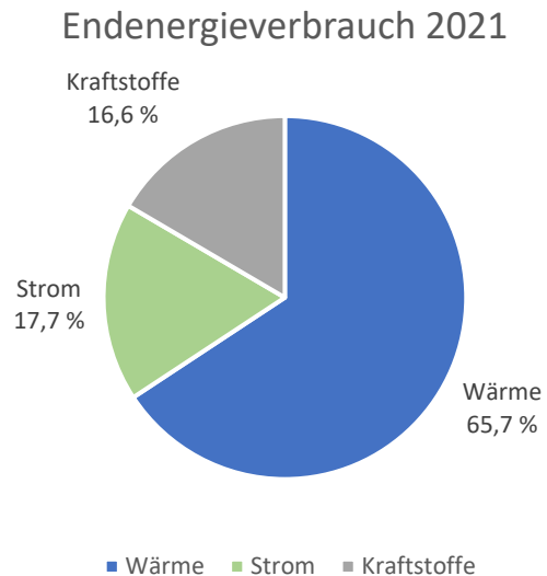
Abbildung 46: Relativer Endenergieverbrauch im Bezirk nach Energieformen und Sekundärenergieträgern . Quelle: Mellon, 2023
