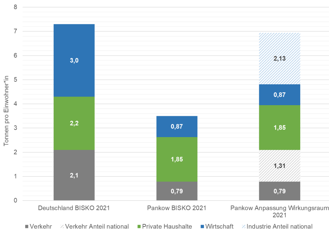
Abbildung 63: Anpassung Wirkungsraum für Restbudgetbestimmung. Quelle: Mellon, 2024
