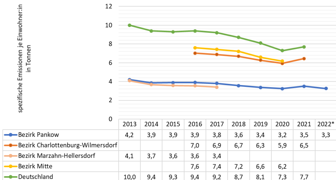
Abbildung 14: spez. THG-Emissionen, Bezirk Pankow im Vergleich zu Deutschland & anderen Bezirken mit BISKO -Bilanz (*vorläufiger Wert). Quelle: Mellon, 2023
