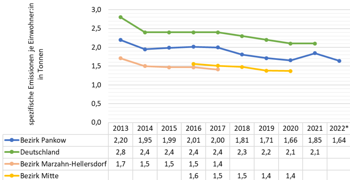
Abbildung 15: spez. THG-Emissionen Sektor Private Haushalte, Bezirk Pankow im Vergleich zu Deutschland & anderen Bezirken (* vorläufiger Wert). Quelle: Mellon, 2023
