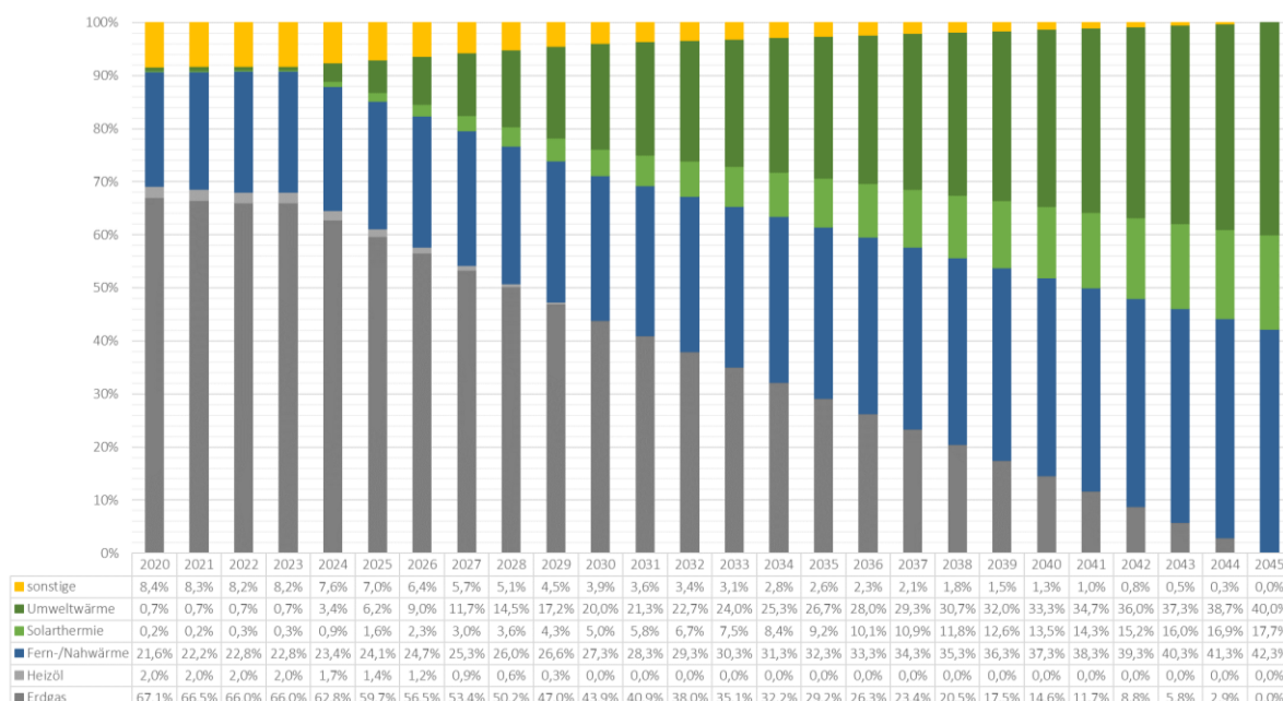
Abbildung 67: Prognose notwendige Entwicklung Wärmemix. Quelle: Mellon, 2024
