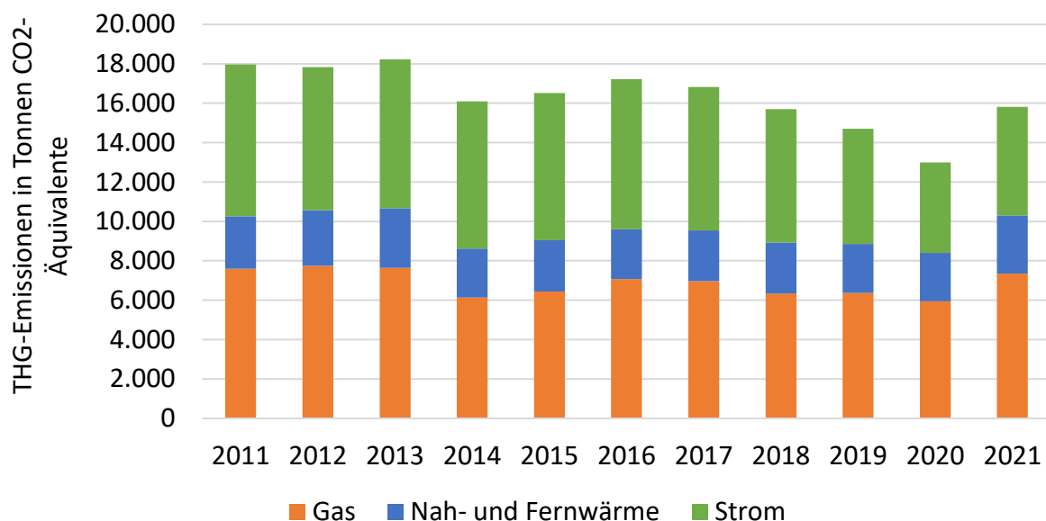
Abbildung 31: THG-Emissionen bezirklicher Gebäude, 2011 – 2021. Quelle: Mellon, 2023
