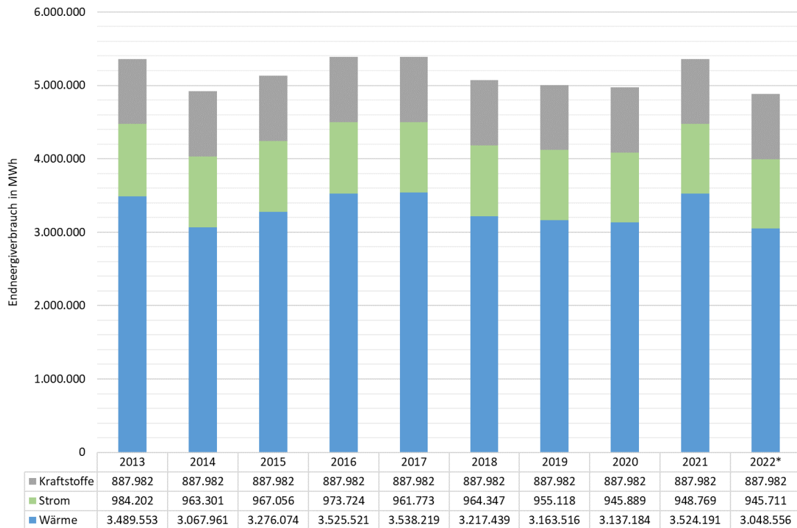
Abbildung 11: Endenergieverbrauch nach Hauptanwendungen; 2013 bis 2022. Quelle: Mellon, 2023
