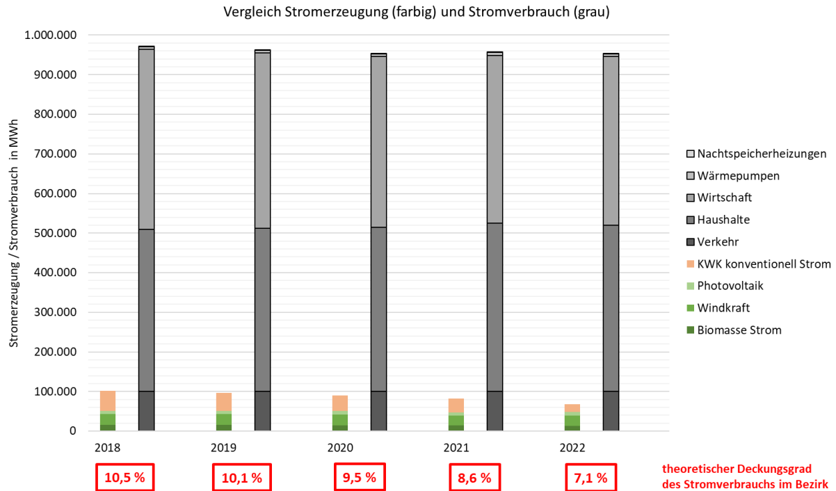
Abbildung 17: Vergleich Stromerzeugung (farbig) und Stromverbrauch (grau). Quelle: Mellon, 2023
