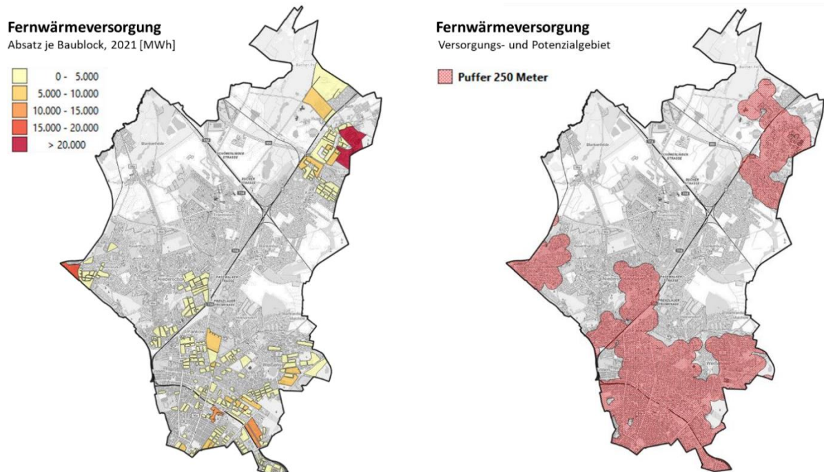
Abbildung 52: Aktueller Status versorgter Baublöcke mit Nah- und Fernwärme und Gebiete im Umkreis um die Wärmenetze. Quelle: Umweltatlas, 2024, eigene Darstellung
