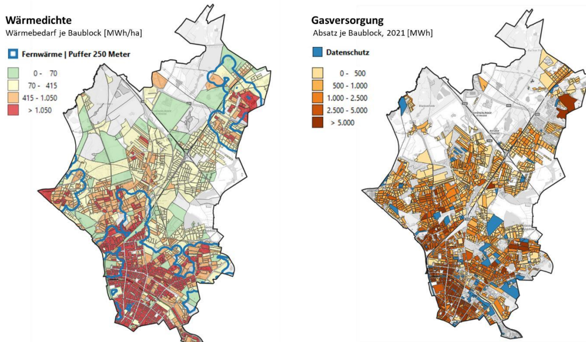
Abbildung 53: Wärmedichte der RBS-Blöcke sowie aktueller Status mit Erdgas versorgter RBS-Blöcke. Quelle: Mellon, 2023
