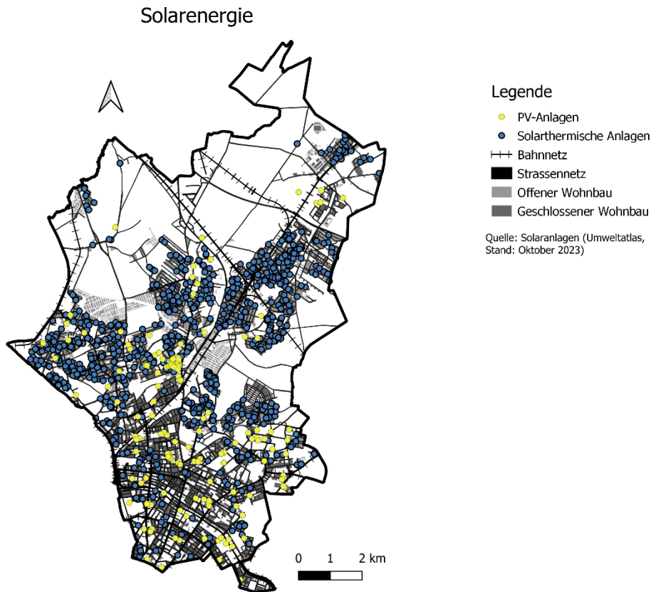
Abbildung 48: Im Bezirk installierte Solaranlagen, Quelle: Umweltatlas, 2024
