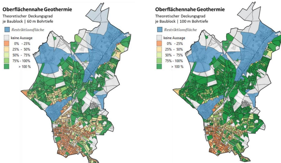
Abbildung 58: Theoretischer Deckungsgrad der Wärmeversorgung durch oberflächennahe Geothermie je Baublock. Quelle: Umweltatlas, Darstellung von Mellon, 2023
