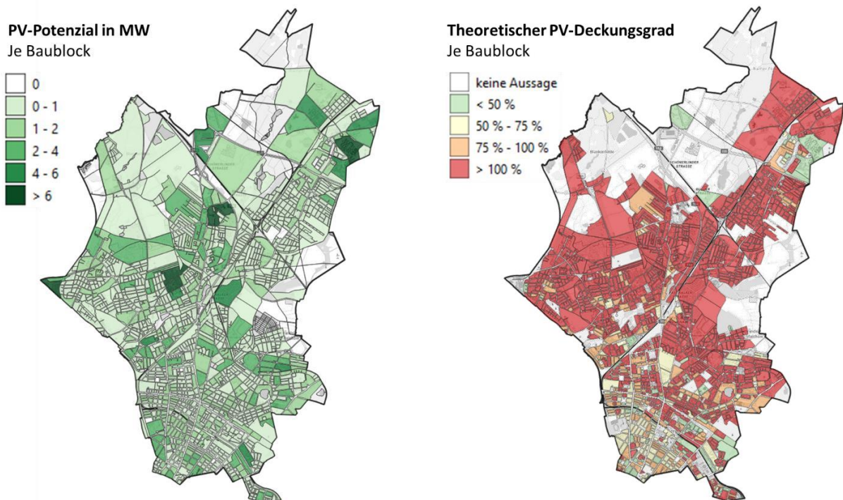
Abbildung 51: Aggregation einzelner Aussagen des PV-Potenzials durch Dachanlagen auf der Ebene von Baublocken. Quelle: Energieatlas, 2024, eigene Darstellung
