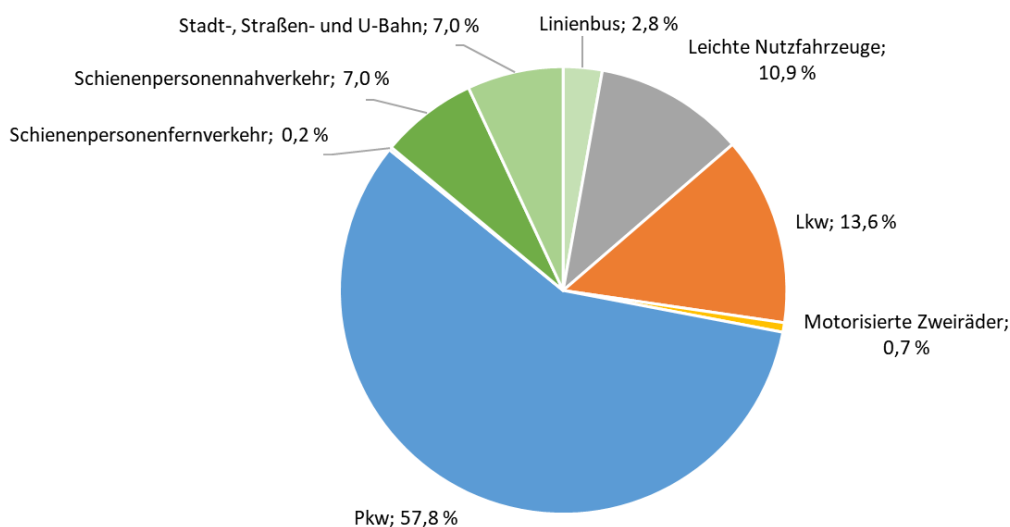
Abbildung 23: Verteilung der THG-Emissionen im Verkehrssektor 2020. Quelle: Mellon, 2023
