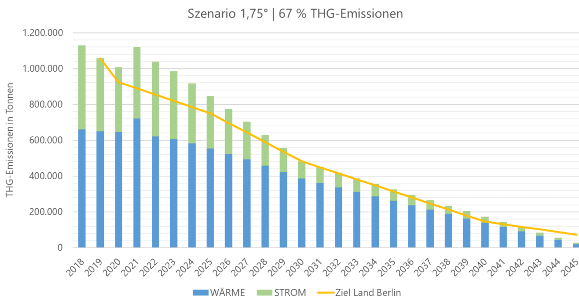
Abbildung 66: Klimaschutzszenario Wärme und Strom unter Beachtung des lokalen Restbudgets (1,75 °C | 67 %) angepasst auf Berliner Ziele. Quelle: Mellon, 2024
