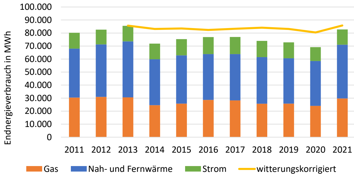
Abbildung 30: Energieverbrauch bezirklicher Gebäude, 2011 – 2021. Quelle: Mellon, 2023
