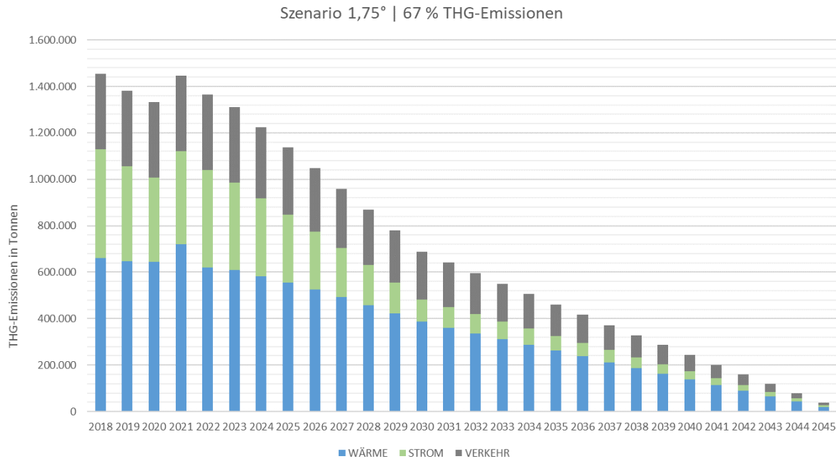
Abbildung 65: Klimaschutzszenario unter Beachtung des lokalen Restbudgets (1,75 °C | 67 %). Quelle: Mellon, 2024
