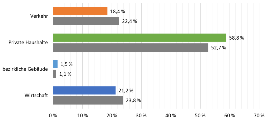
Abbildung 12: Anteile der Sektoren am Endenergieverbrauch und THG-Emissionen – 2021. Quelle: Mellon, 2023
