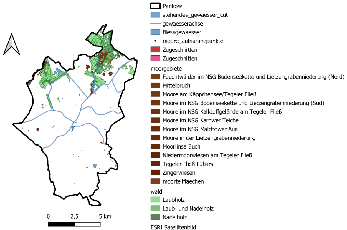
Abbildung 24: Wald- und Moorflächen Pankow. Quelle: Umweltatlas, 2024, eigene Darstellung
