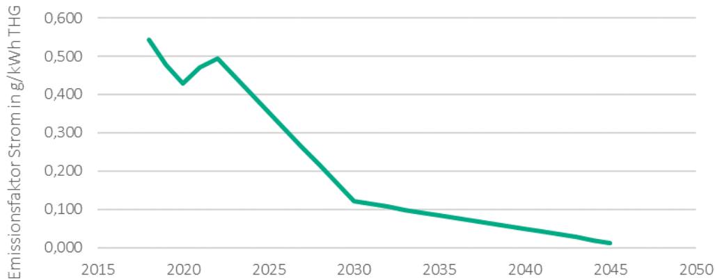
Abbildung 68: Prognose Strommix Deutschland Emissionsfaktor auf Basis Zielstellungen bundesweit. Quelle: Mellon, 2024
