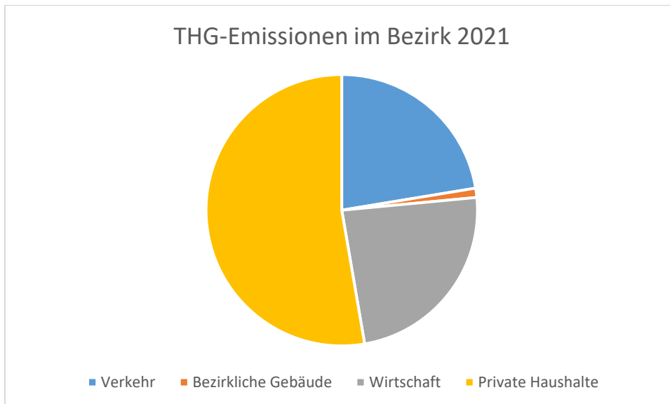
Abbildung 44: Relative THG-Emissionen in Bezirk Pankow 2021 nach Sektoren. Quelle: Mellon, 2023
