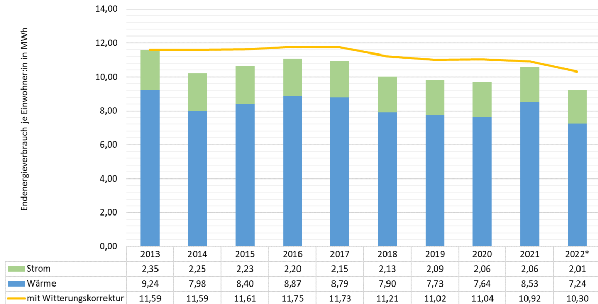
Abbildung 10: Endenergieverbrauch stationär pro Einwohner:in; 2013 bis 2022 (*2022 nur als vorläufiger Wert). Quelle: Mellon, 2023
