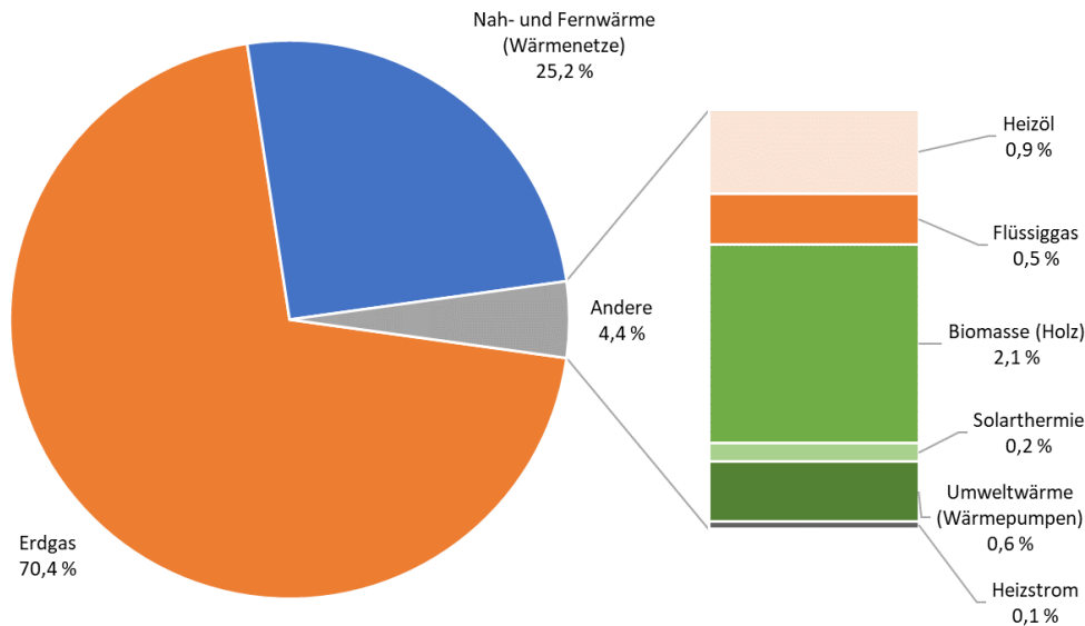
Abbildung 19: Anteile am Energieverbrauch im Wärmemix der Wirtschaft 2021. Quelle: Mellon, 2023
