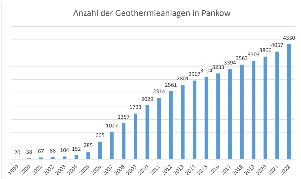
Abbildung 50: Anzahl der durch den Energieatlas Berlin erfassten Geothermieranlagen im Bezirk Pankow. Quelle, Energieatlas, 2024
