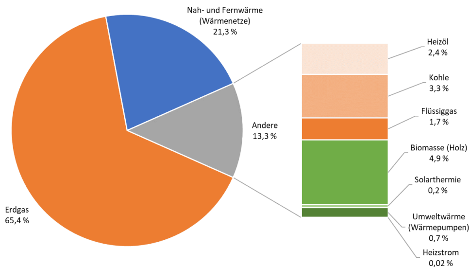
Abbildung 18: Anteile am Energieverbrauch im Wärmemix der Haushalte 2021. Quelle: Mellon, 2023
