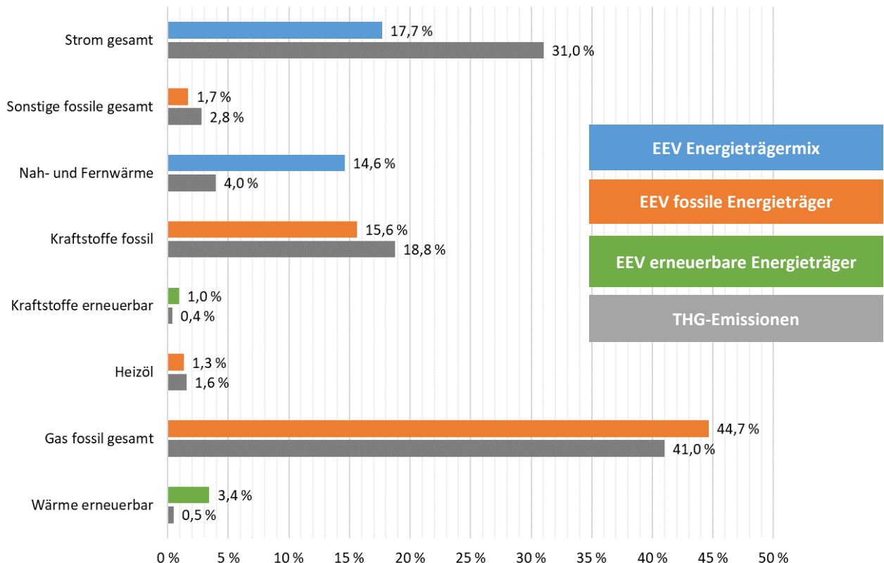
Abbildung 13: Anteile der Energieträger am Endenergieverbrauch und THG-Emissionen – 2021. Quelle: Mellon, 2023
