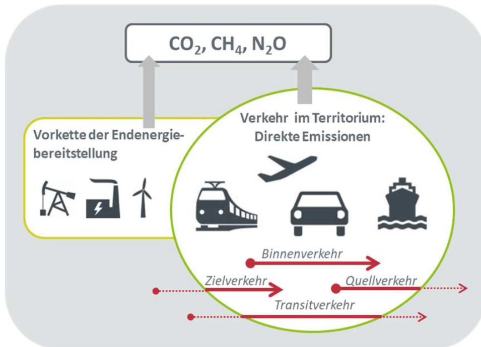
Abbildung 89: BISCO-Prinzip im Sektor Verkehr, Quelle: ifeu 2019
