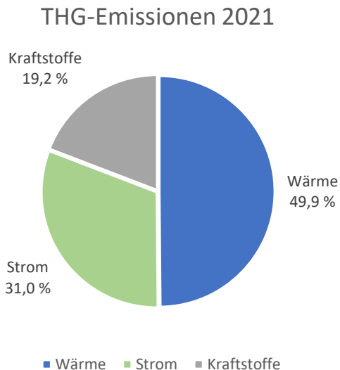
Abbildung 45: Relative THG-Emissionen im Bezirk Pankow nach Energieformen und Sekundärenergieträgern . Quelle: Mellon, 2023
