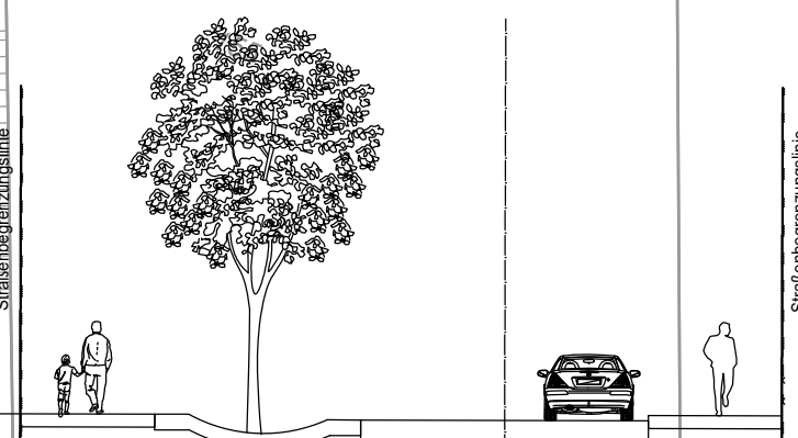
geplanter Querschnitt Ferdinand-Buisson-Straße von Ludwig-Quide-Straße bis Haus-Nr. 31A M 1:100
