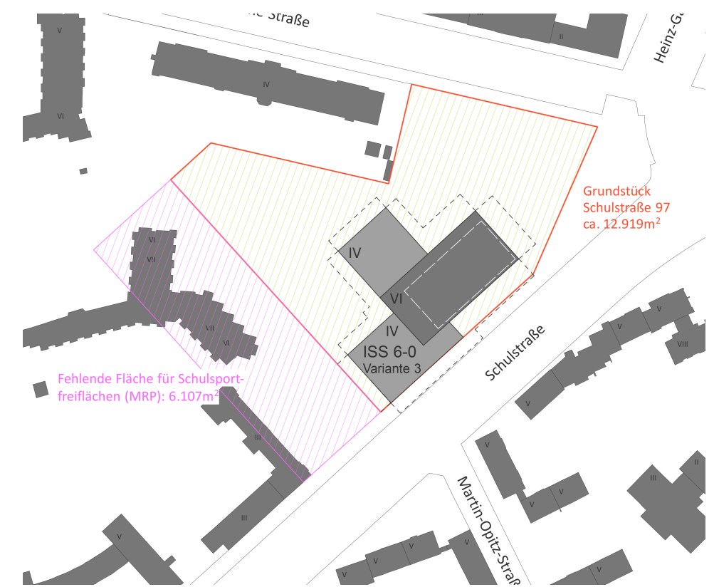
Lageplan ISS 6-0, Bauungsvariante 3 (alle © S.T.E.R.N. GmbH, Grundlage: Geoportal Berlin / Berliner Vermessungsämter)
