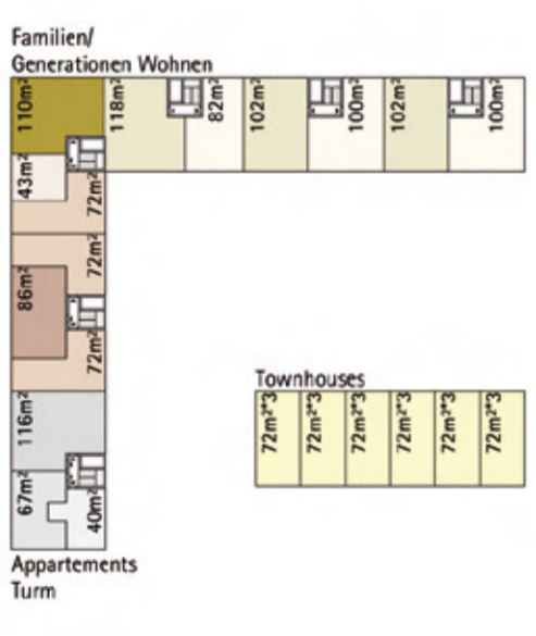
Variante 2 Fokus: mittlere WE hier: 100 WE (40-116m²)
