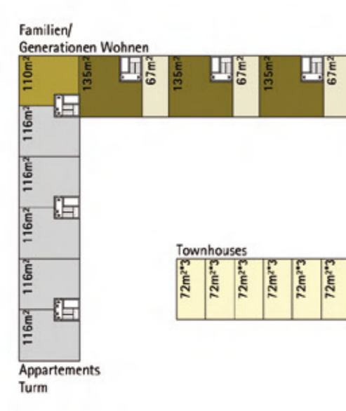
Variante 3 Fokus: große WE hier: 84 WE (60-135m²)
