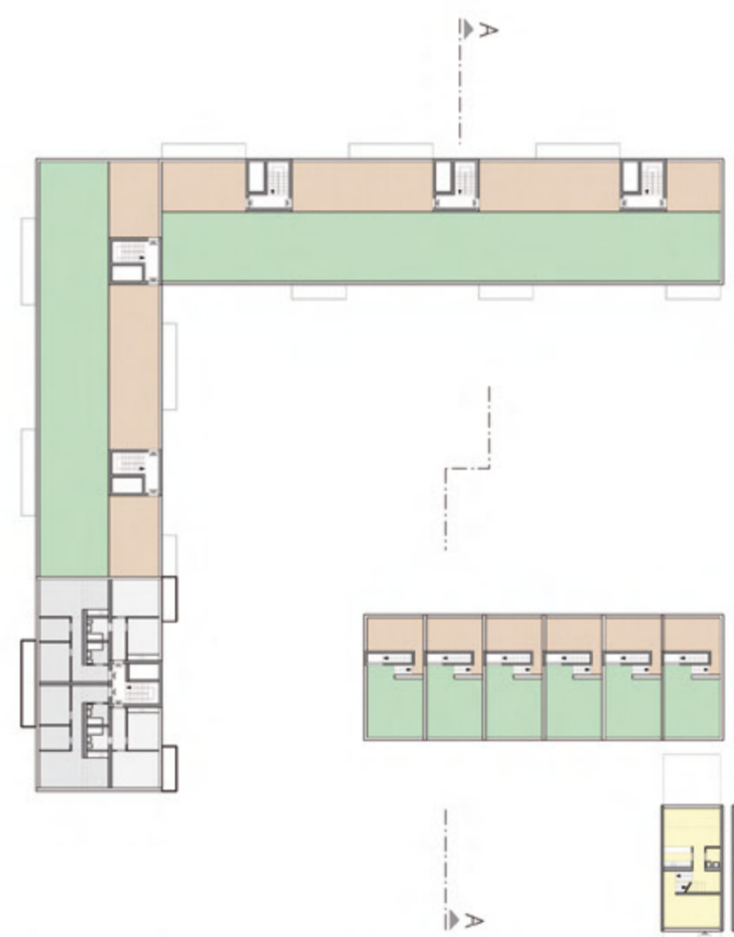
Grundriss Dachgeschoss M 1:500
