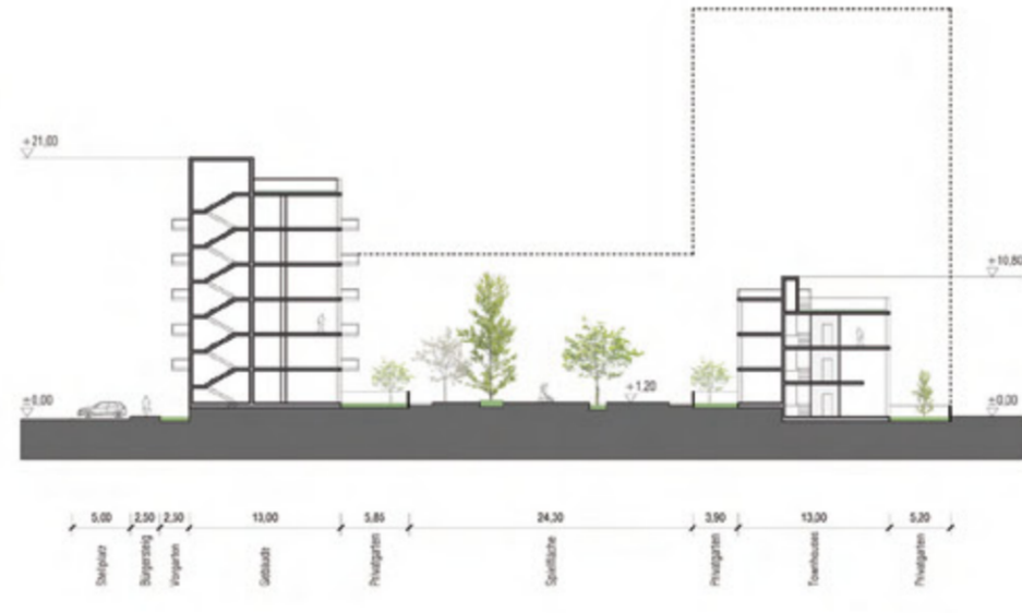
Schnitt
