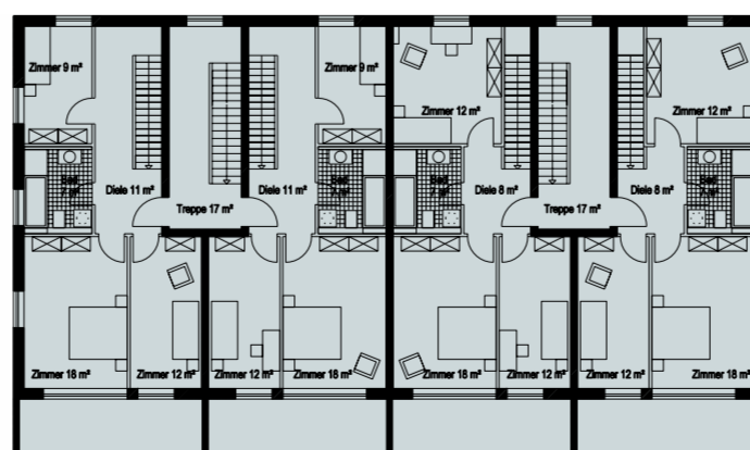
3. Obergeschoss 57m 2 Wohnfläche 3. Obergeschoss 57m 2 Wohnfläche 3. Obergeschoss 57m 2 Wohnfläche 3. Obergeschoss 57m 2 Wohnfläche
