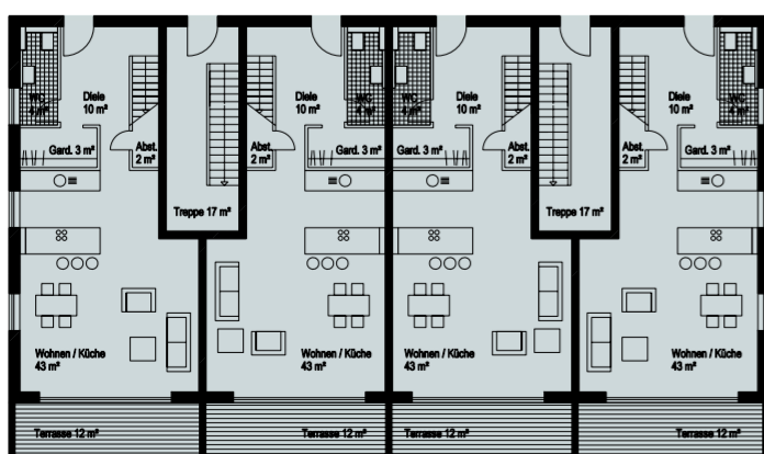
2. Obergeschoss 68m 2 Wohnfläche 2. Obergeschoss 68m 2 Wohnfläche 2. Obergeschoss 68m 2 Wohnfläche 2. Obergeschoss 68m 2 Wohnfläche
