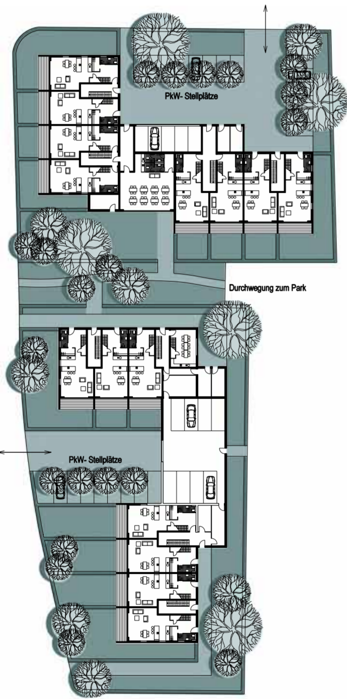
Erdgeschoss M 1:500
