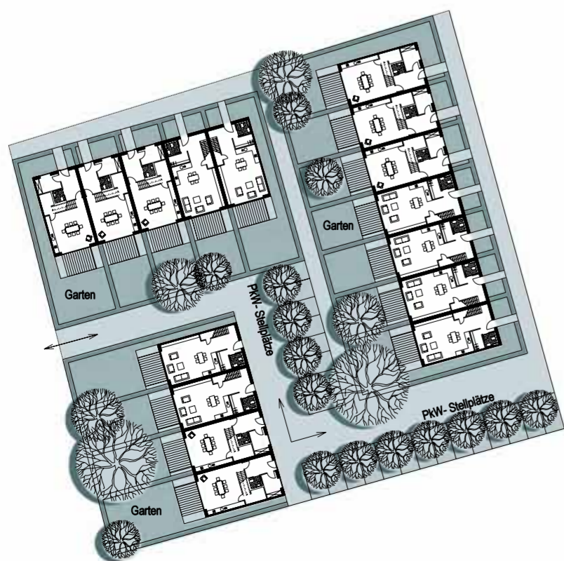
Erdgeschoss M 1:500
