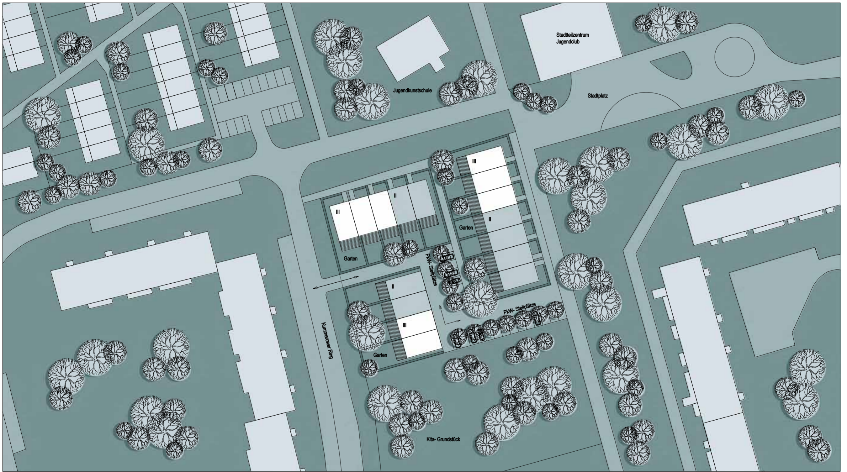
Lageplan M 1:500
