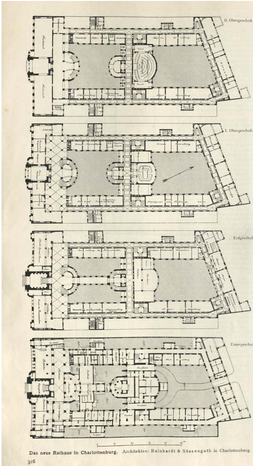
Grundriss des preisgekrönten Entwurfs von Reinhardt & Süßenguth, im damaligen 1. OG ist die Bibliothek eingezeichnet. Deutsche Bauzeitung, 1904, S. 316.
