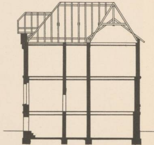
SCHNITT A-B.
