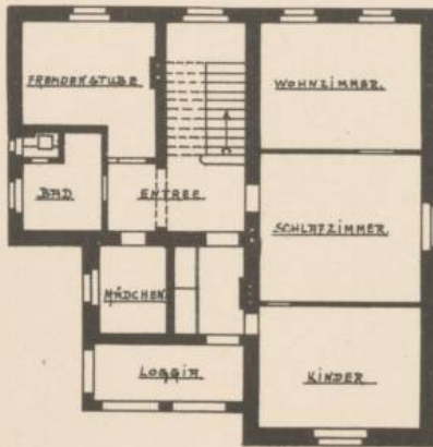
ERSTES STOCKWERK.
