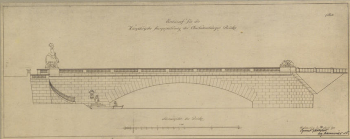
Querschnitt.
