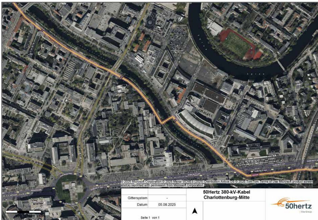
Abb. 53: Leitungsplan der 50 Hertz GmbH, Quelle: 50 Hertz GmbH
