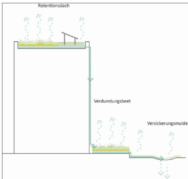
Abb. 47: Schematische Kaskade der Regenwasserbewirtschaftung für Baufeld mit Verdunstung/Versickerung im Hof, Quelle: bgmr (Abbildung)
