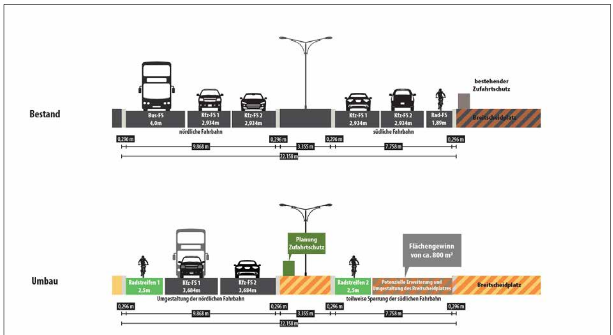
Abb. 62: Querschnitt Budapester Straße (vorm Bikini-Haus) Bestand (oben) und Umgestaltungsvorschlag, Quelle: Büro Happold
