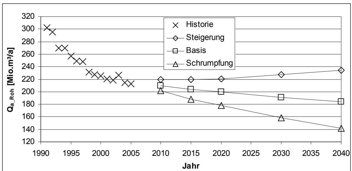
Abb. 15: Jährliche Rohwasserrförmengen von 1991 bis 2005 und deren Prognose für die Varianten Basis, Steigerung und Schrumpfung.
