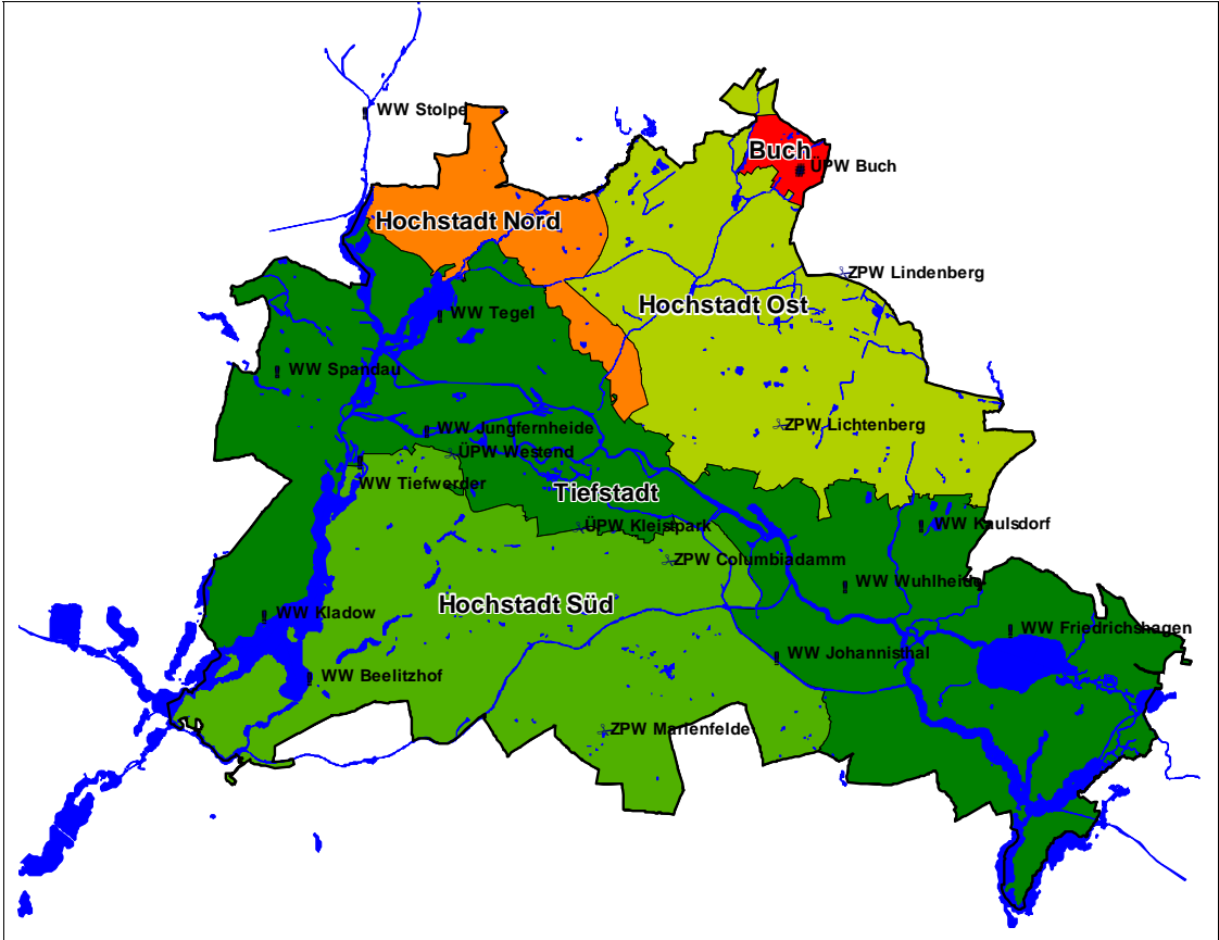
Abb. 3: Druckzonen der Trinkwasserverteilung in Berlin (Quelle: BWB).
