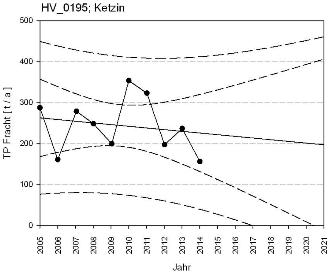
Abbildung 4 Entwicklung der Gesamtposphat-Fracht in der Havel bei Ketzin in den Jahren 2005 – 2014, Abschätzung des Trends (—) und der wahrscheinlichen Entwicklung des Trends (inneres Band - -, 95% Vertrauensintervall) und der Jahresmittelwerte (äußeres Band - -, 95% Vertrauensintervall) bis zum Jahr 2021.
