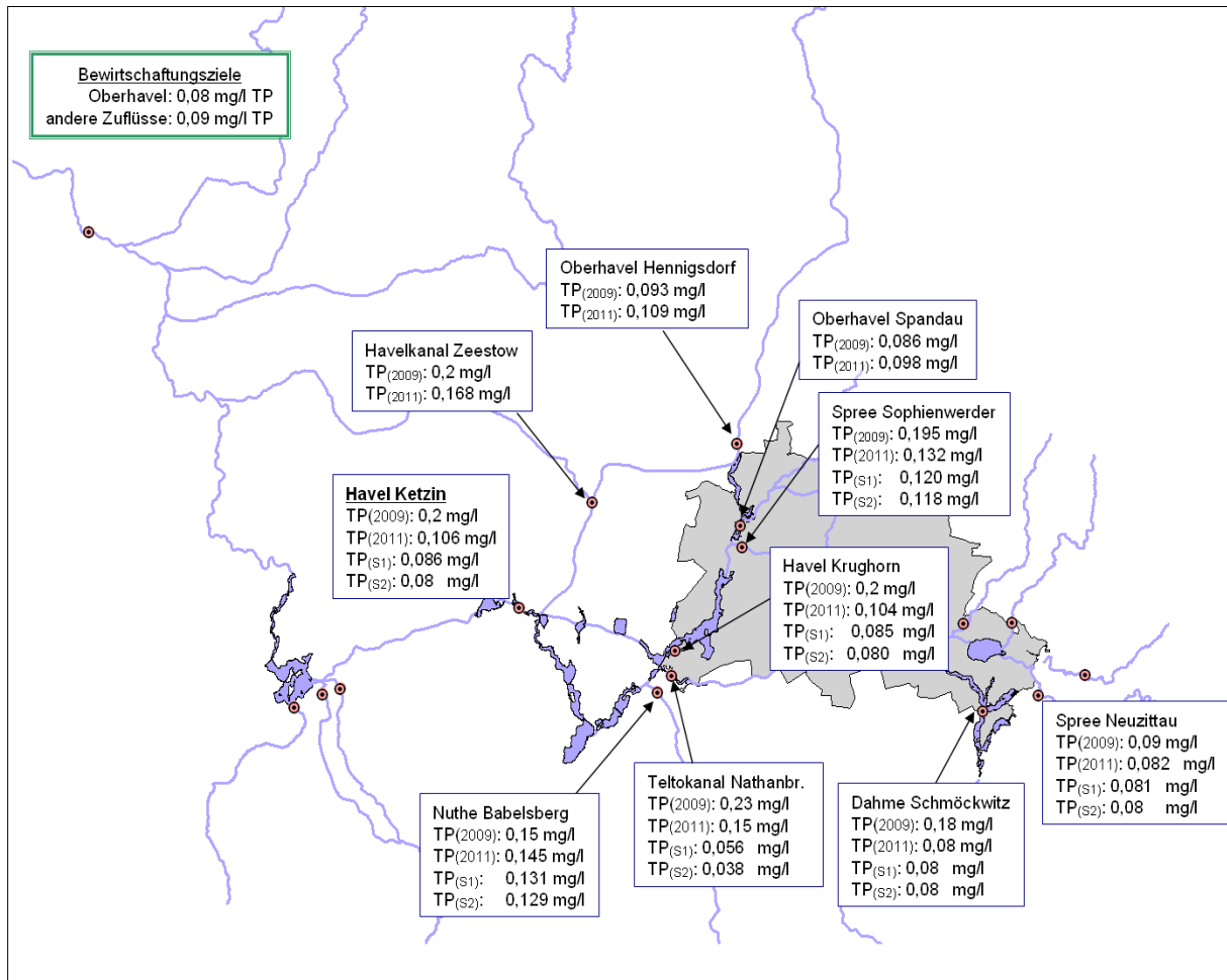
Abbildung 8: Prognostizierte TP-Konzentrationen an wichtigen Messstellen im Wirkungsraum des Nährstoffreduzierungskonzeptes durch Maßnahmen an Großklärwerken ( TP_{(2009)} = Mittelwert Gesamtposphor 2009, TP_{(2011)} = Mittelwert Gesamtposphor 2011, TP_{(S1)} =Szenario 1, TP_{(S2)} =Szenario 2).
