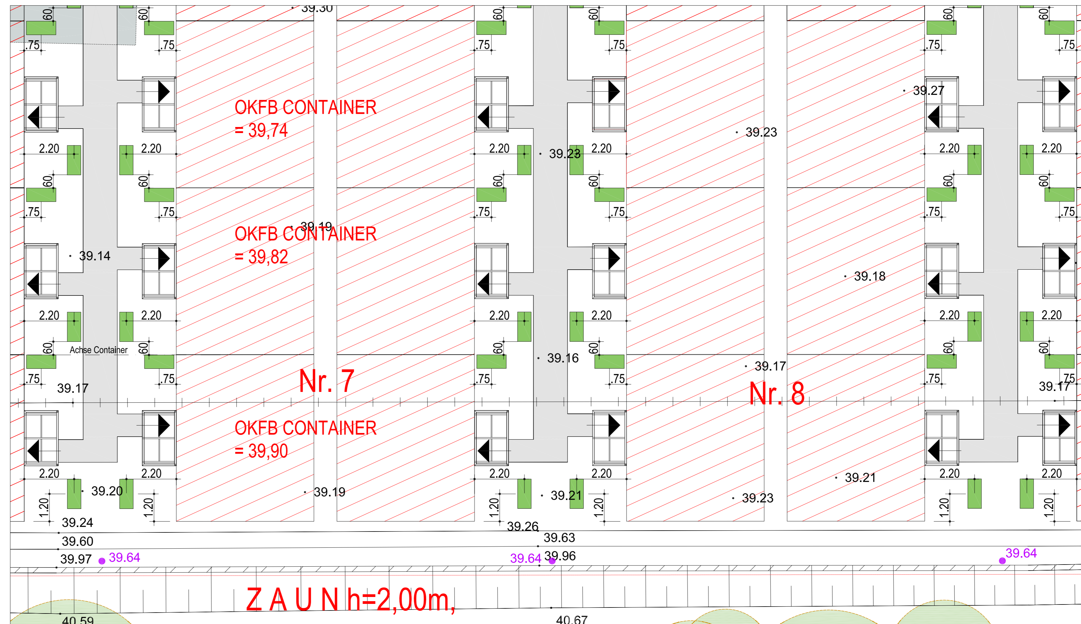
AUSZUG_Anordnung Hochbeete_Containerreihe 7_M 1:100
