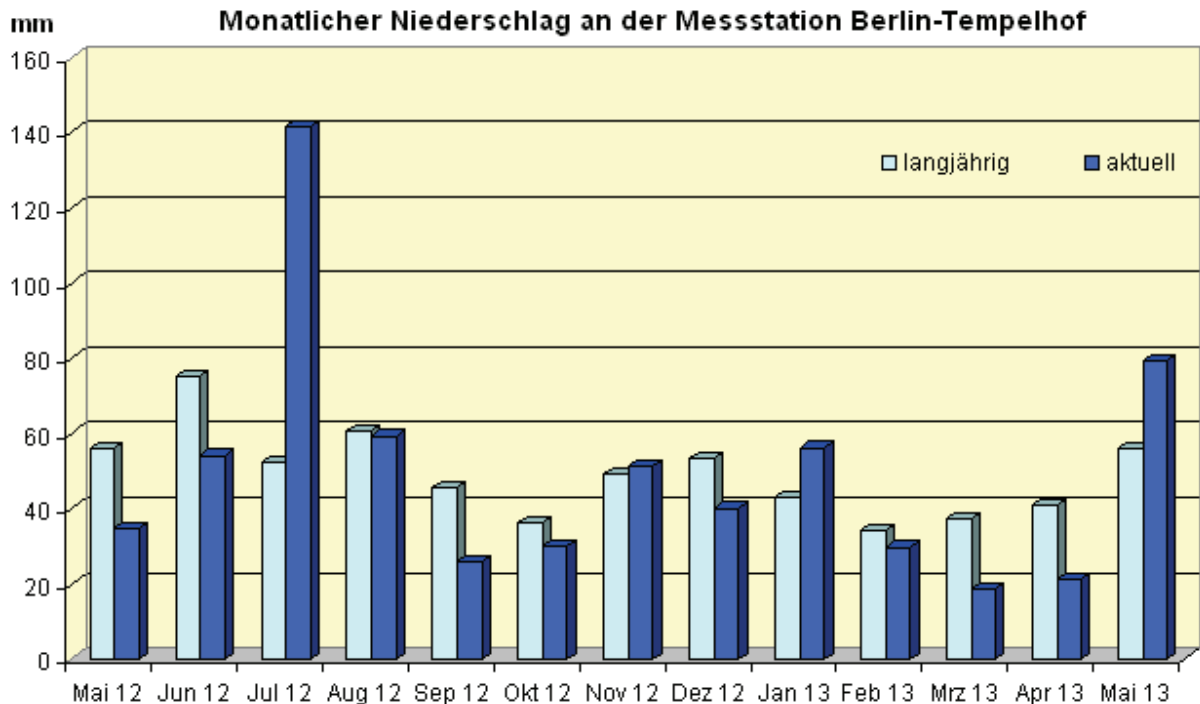
Abb. 15: Monatlicher Niederschlag von Juni 2012 bis Mai 2013 der Messstation Berlin-Tempelhof im Vergleich mit dem langjährigen Mittel 1961 bis 1990
