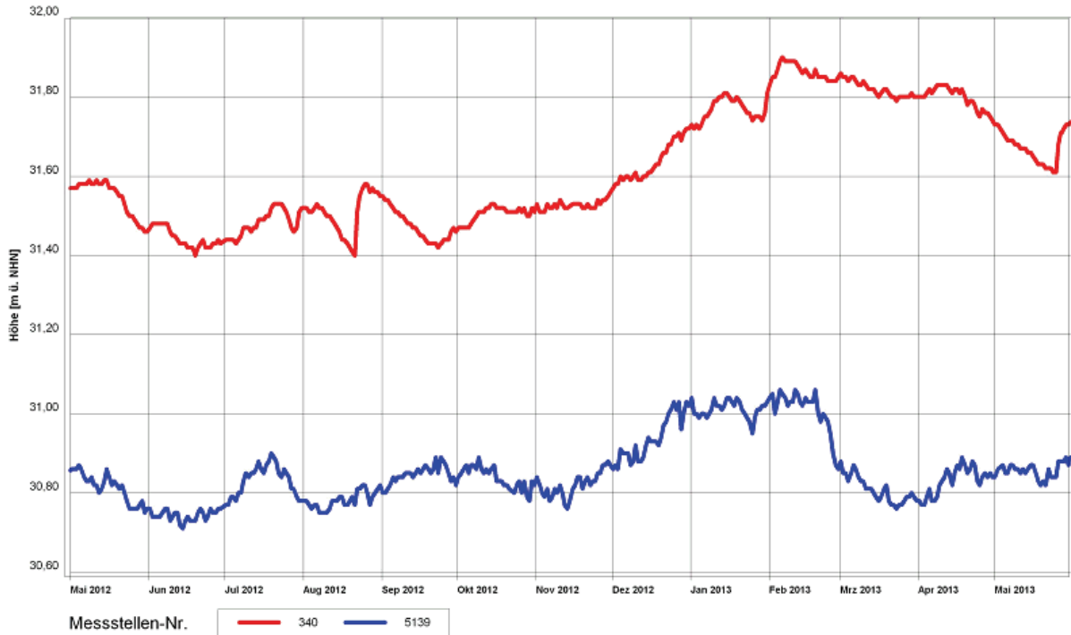
Abb. 13: Grundwasserstandsganglinien von zwei beispielhaften Messstellen im Urstromtal von Mai 2012 bis Mai 2013
