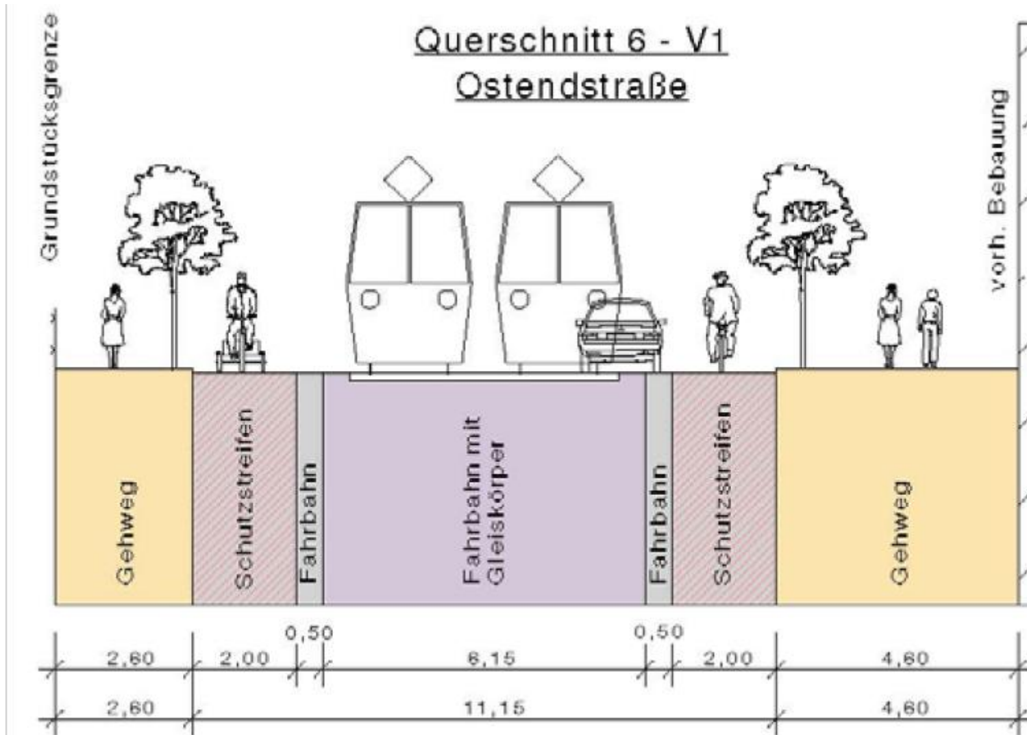
Querschnitt Planung, Quelle: Machbarkeitsstudie 2011
