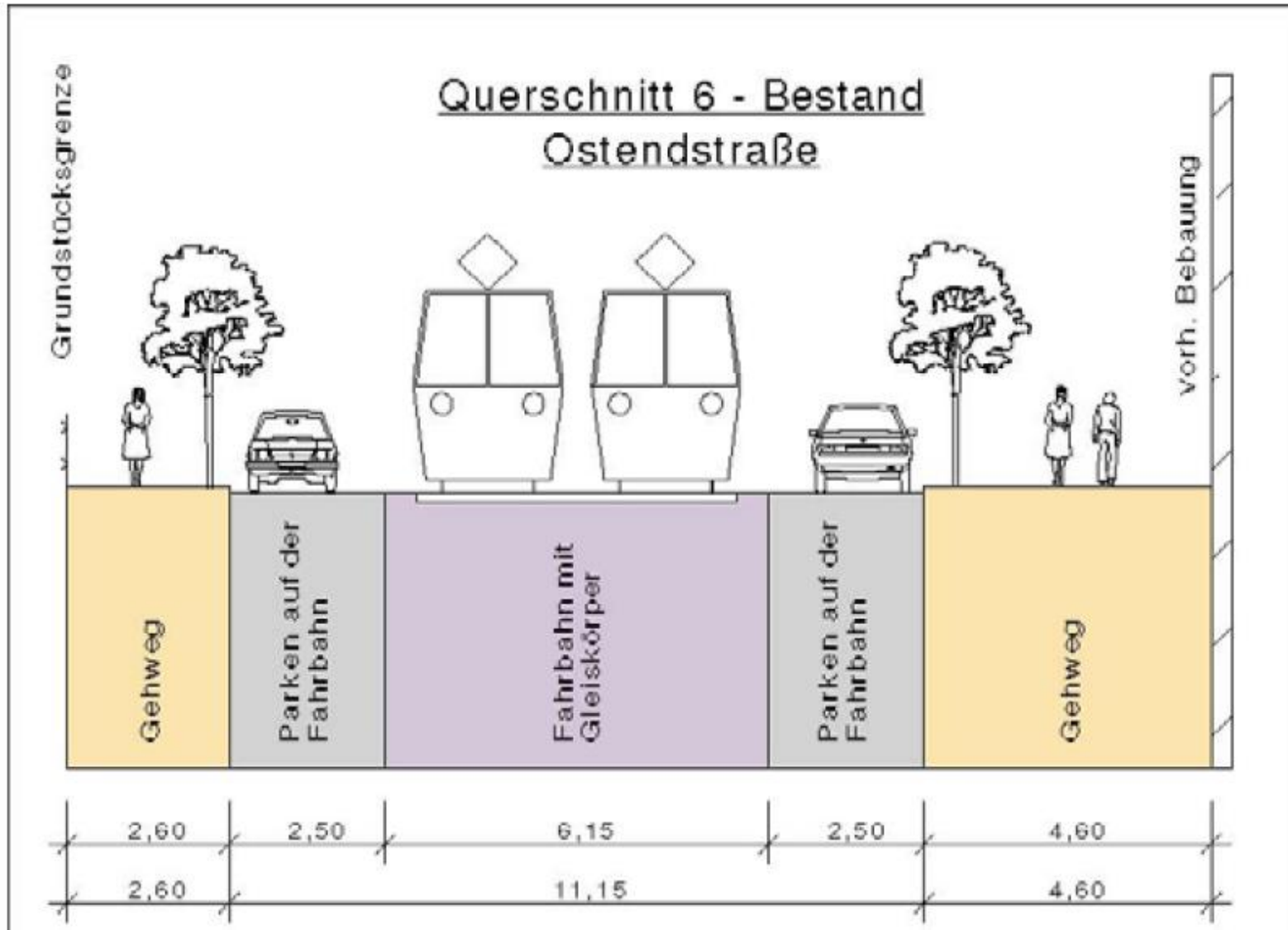
Querschnitt Bestand, Quelle: Machbarkeitsstudie 2011
