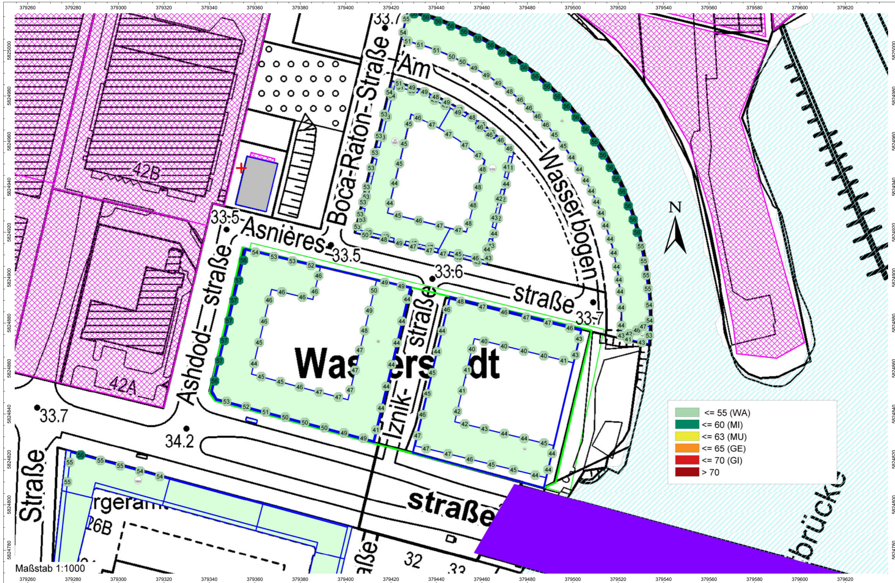
Gebäudelärmkarte: Beurteilungspegel Lr in dB(A), höchster Fassadenpegel Szenario: Gewerbelärm; Ersatzschallquellen; mit exemplarischem Baukörperentwurf - TAGZEIT 6-22 Uhr M166931/02 jgr Mai 2023
