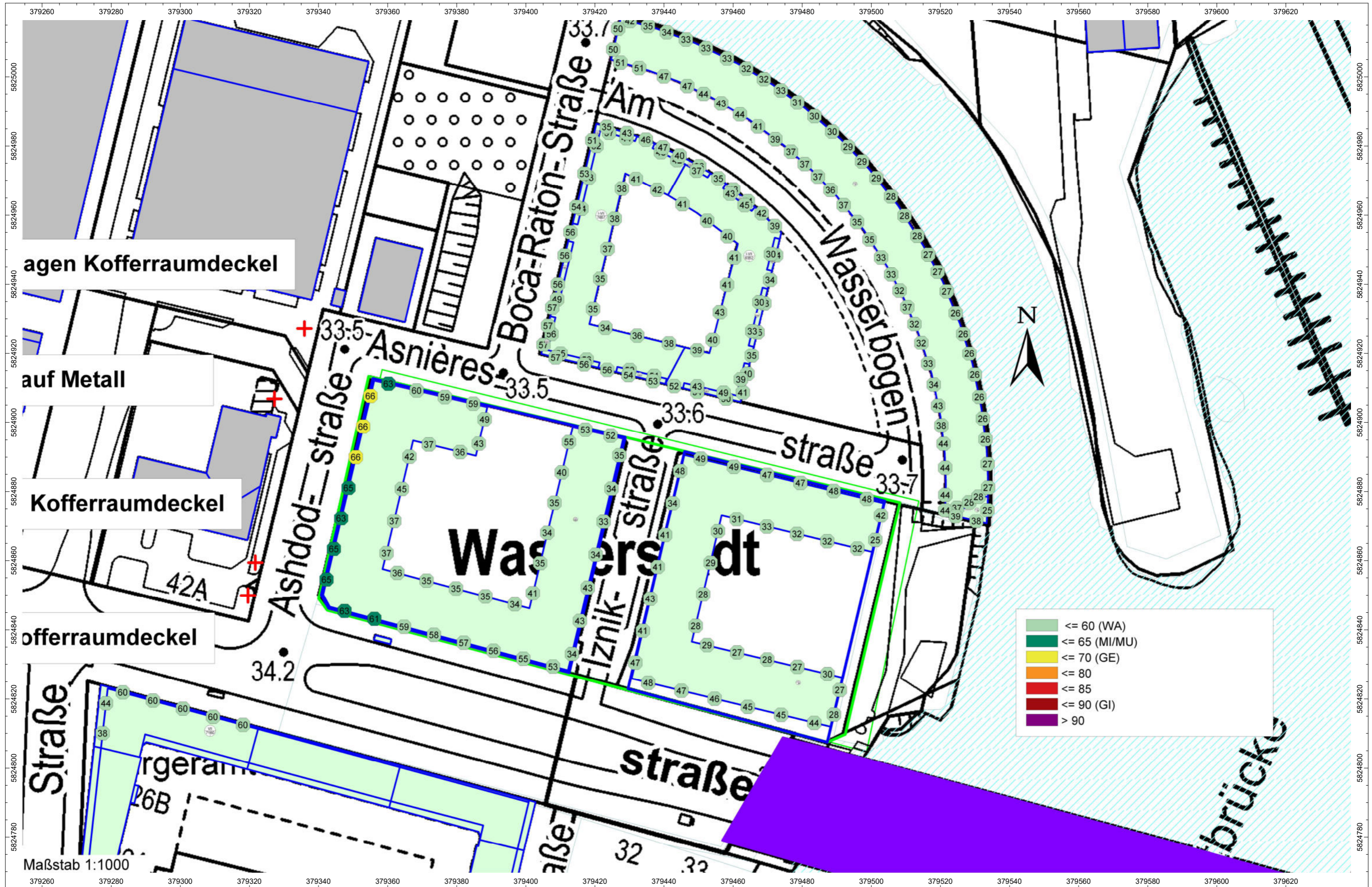
Gebäudelärmkarte: Kurzzeitige Geräuschspitzen L_AFmax Lr in dB(A), höchster Fassadenpegel, höchster Pegel aus den 4 Quellpositionen Szenario: Gewerbelärm - Kurzzeitige Geräuschspitzen; mit exemplarischem Baukörperentwurf - NACHT 22-6 Uhr
