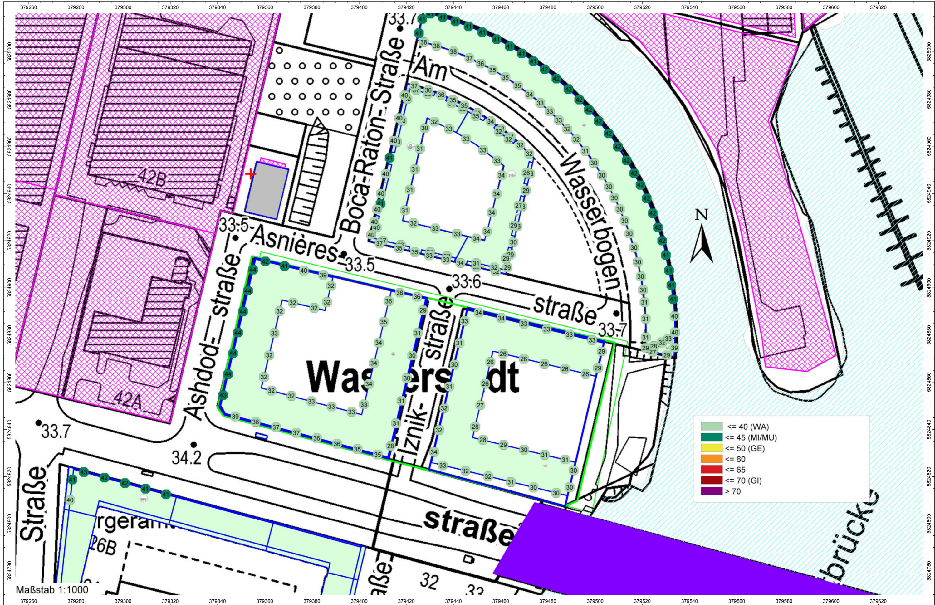
Gebäudelärmkarte: Beurteilungspegel Lr in dB(A), höchster Fassadenpegel Szenario: Gewerbelärm; Ersatzschallquellen; mit exemplarischem Baukörperentwurf - lauteste NACHTstunde 22-6 Uhr
