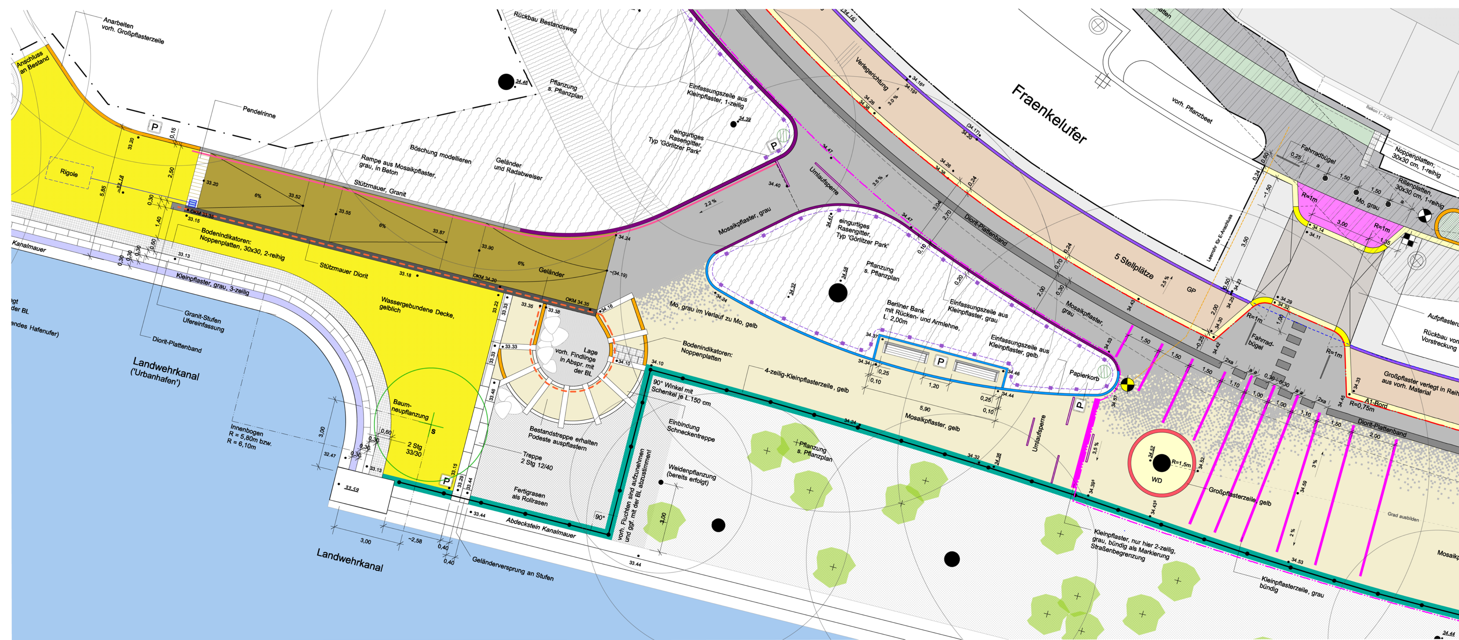
Ausschnitt Bereich Urbanhafen M 1:100
